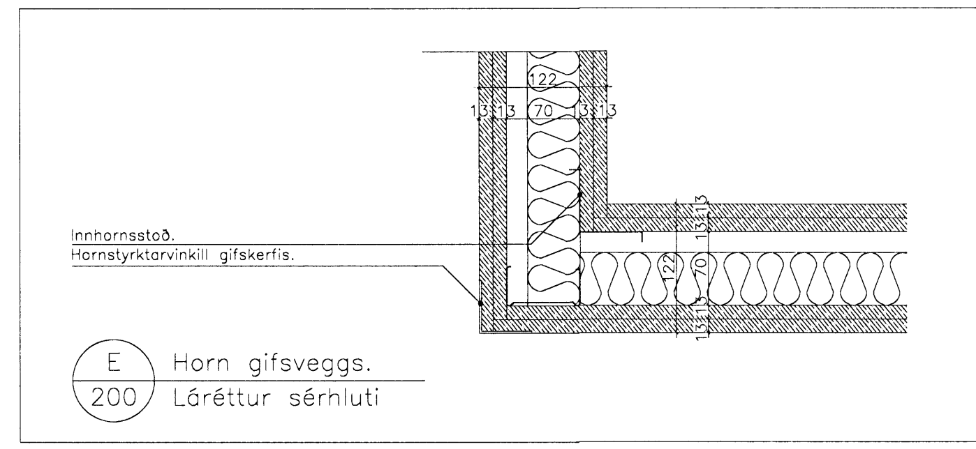
F Horn gífsveggis. 204 Láréttur sérhluti
