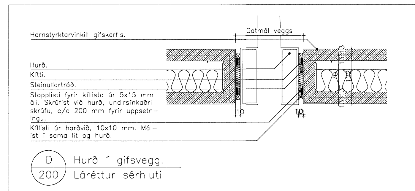
E Horn gífsveggis. 200 Láréttur sérhluti
