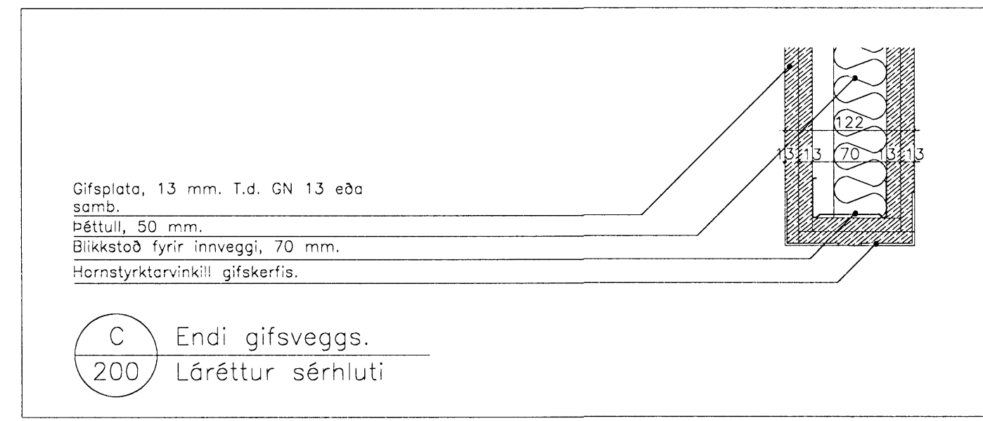
D Hurð í gífsvegg. 200 Láréttur sérhluti
