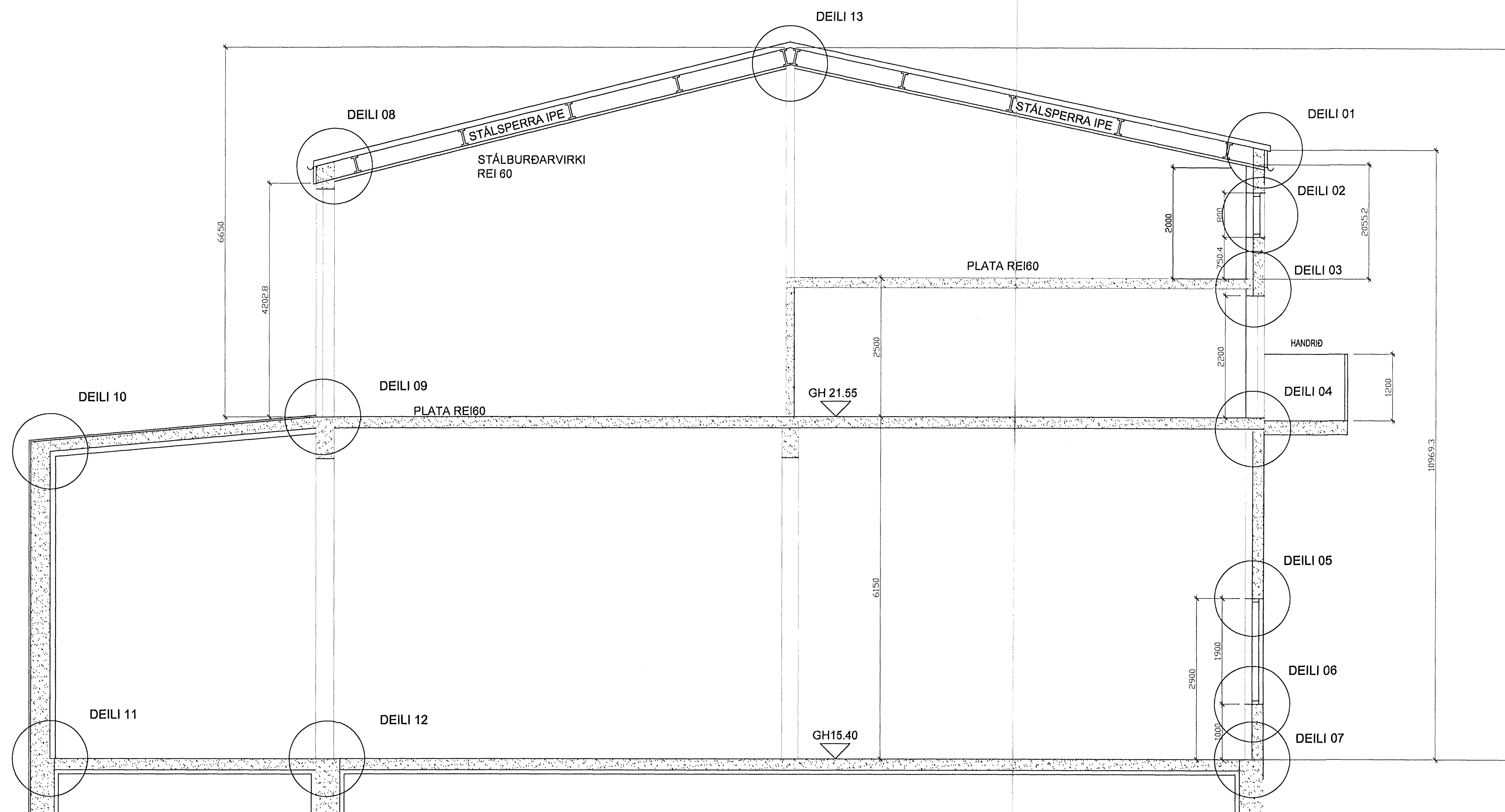
SNID A-A 1:50
