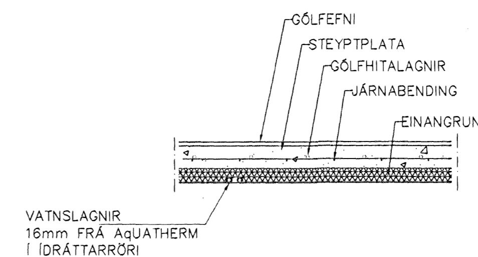
LAGNIR, SNIÐ, 1:20
