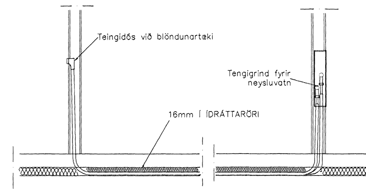
TENING NEYSLUVATNSLAGNA 1:20
