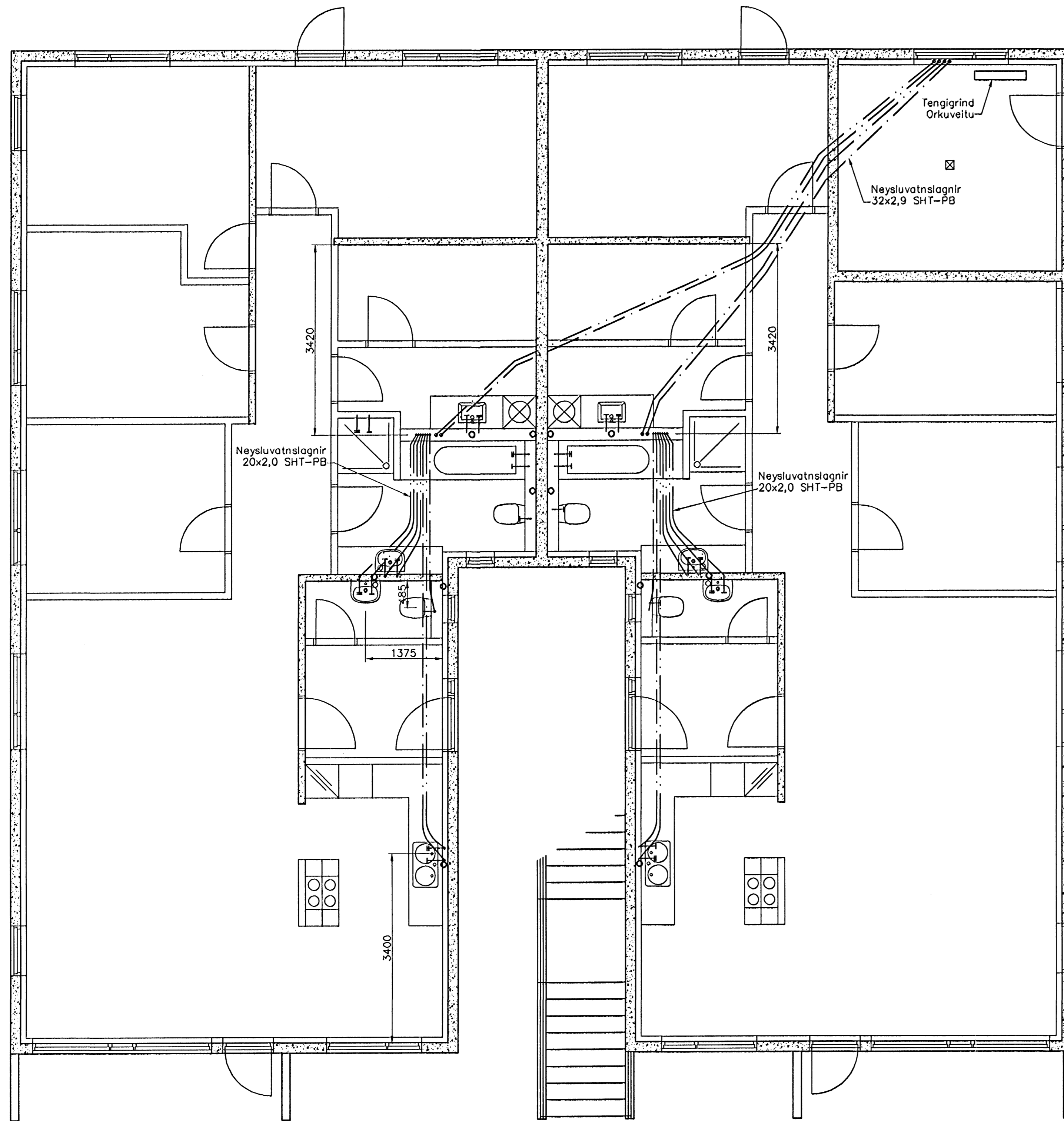
Stofnlaginir, Grunnmynd, 1:50
