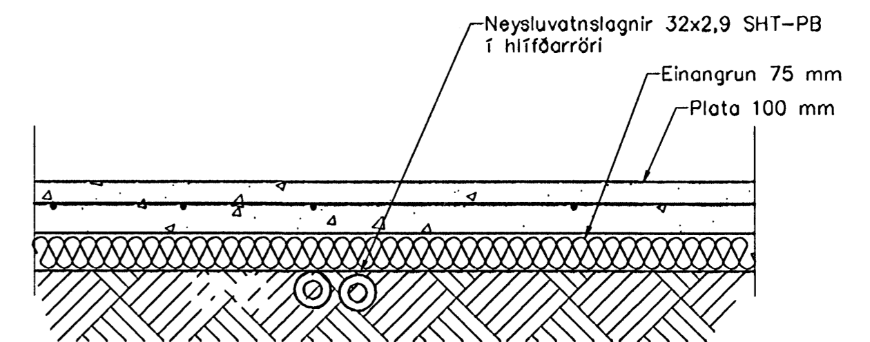
Hita- og Neysluvatnslagnir, Snið í botnplötu, 1:10
