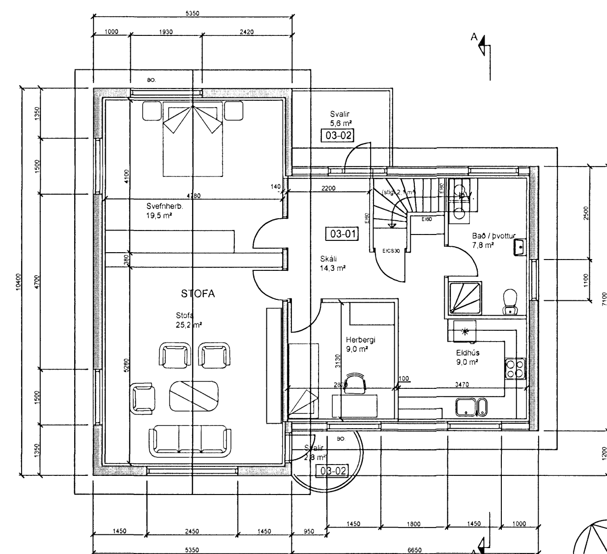
Grunnmynd 3.Hæðar 1:100
