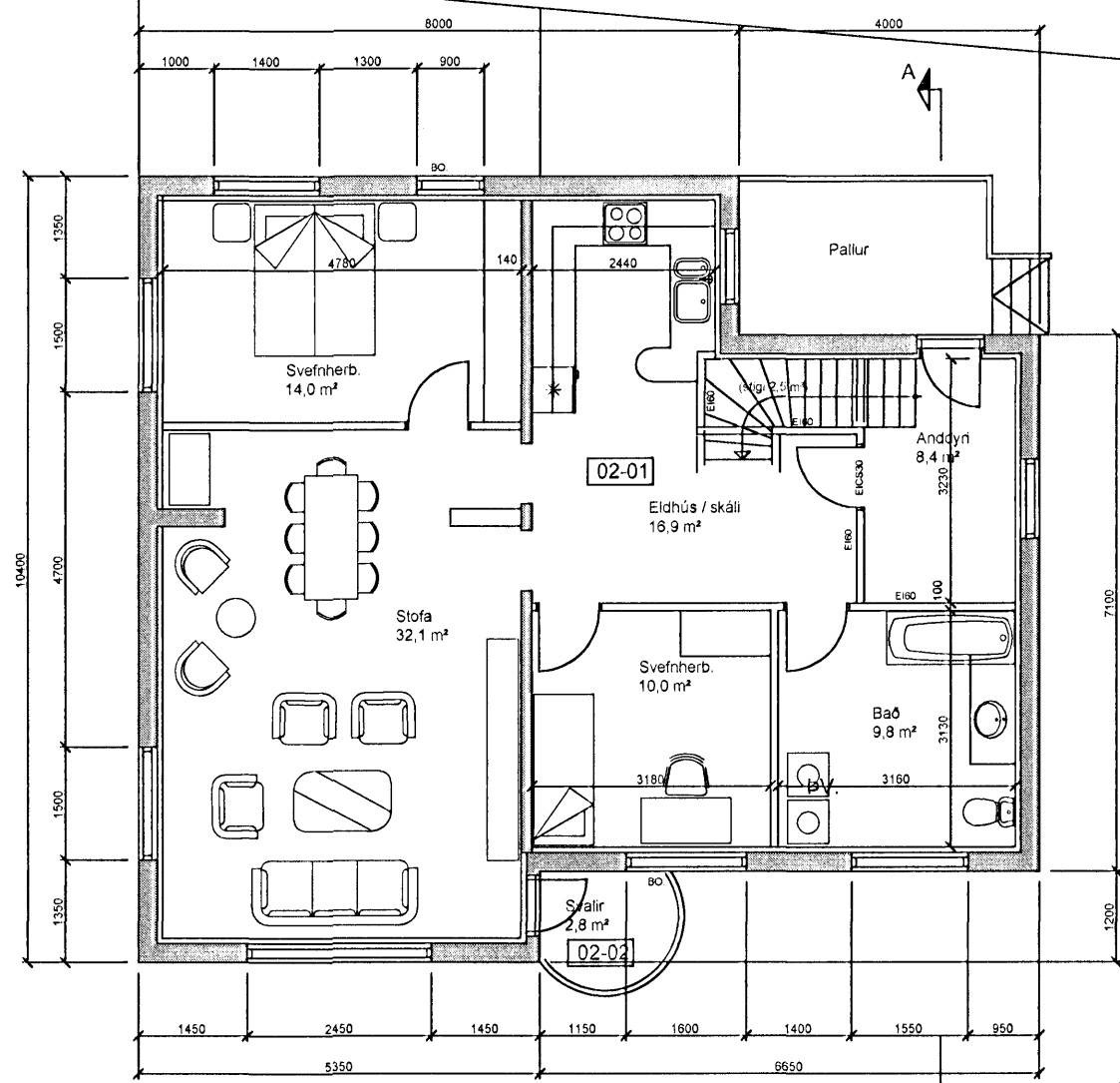
Grunnmynd 2.Hæðar 1:100
