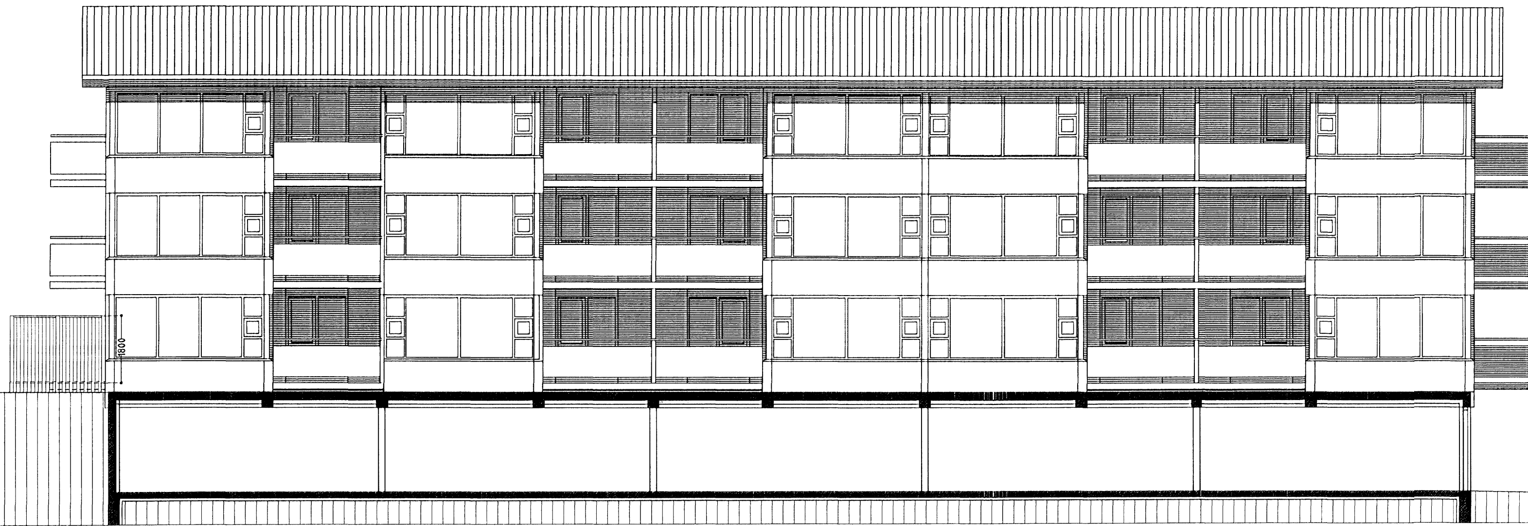
ÚTLIT SUÐ-AUSTUR. mkv. 1:100.
