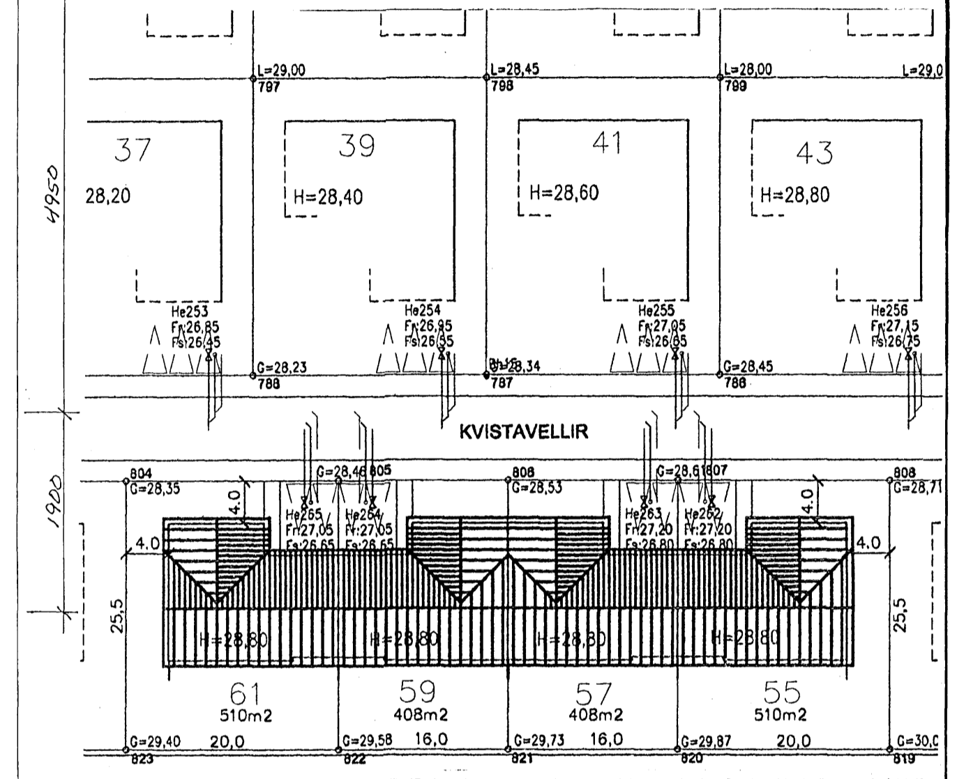
Afstöðumynd M = 1:500
