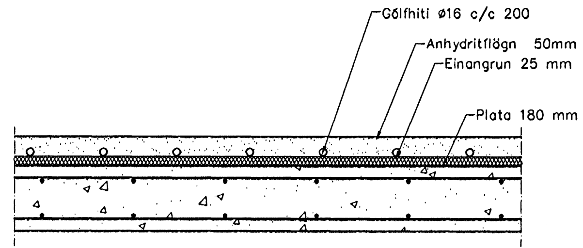
Gólfhiti, Snið í milliþötu, 1:10
