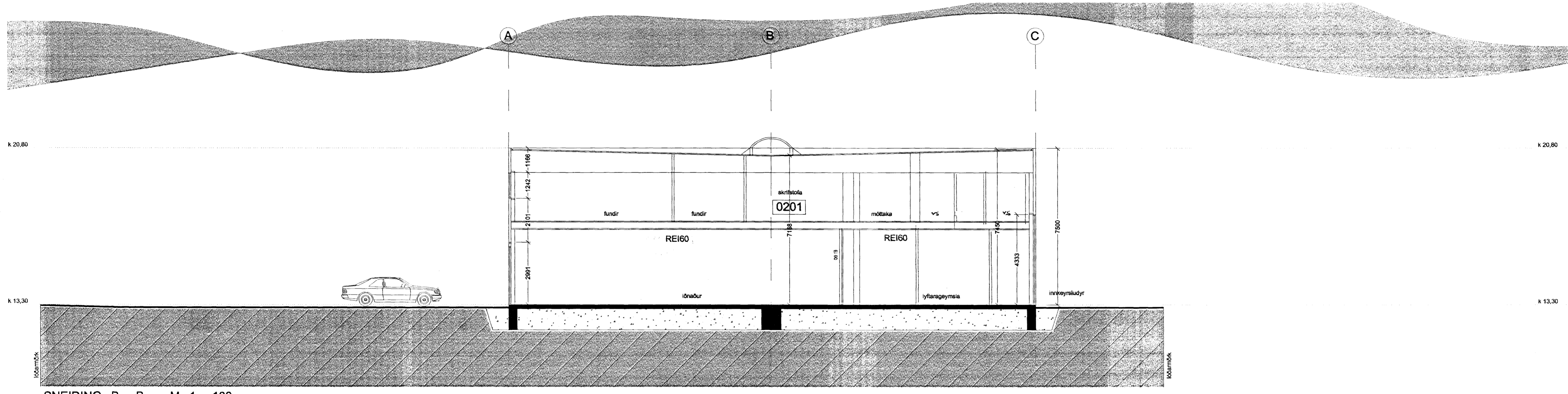
SNEIÐING B - B M 1 : 100
