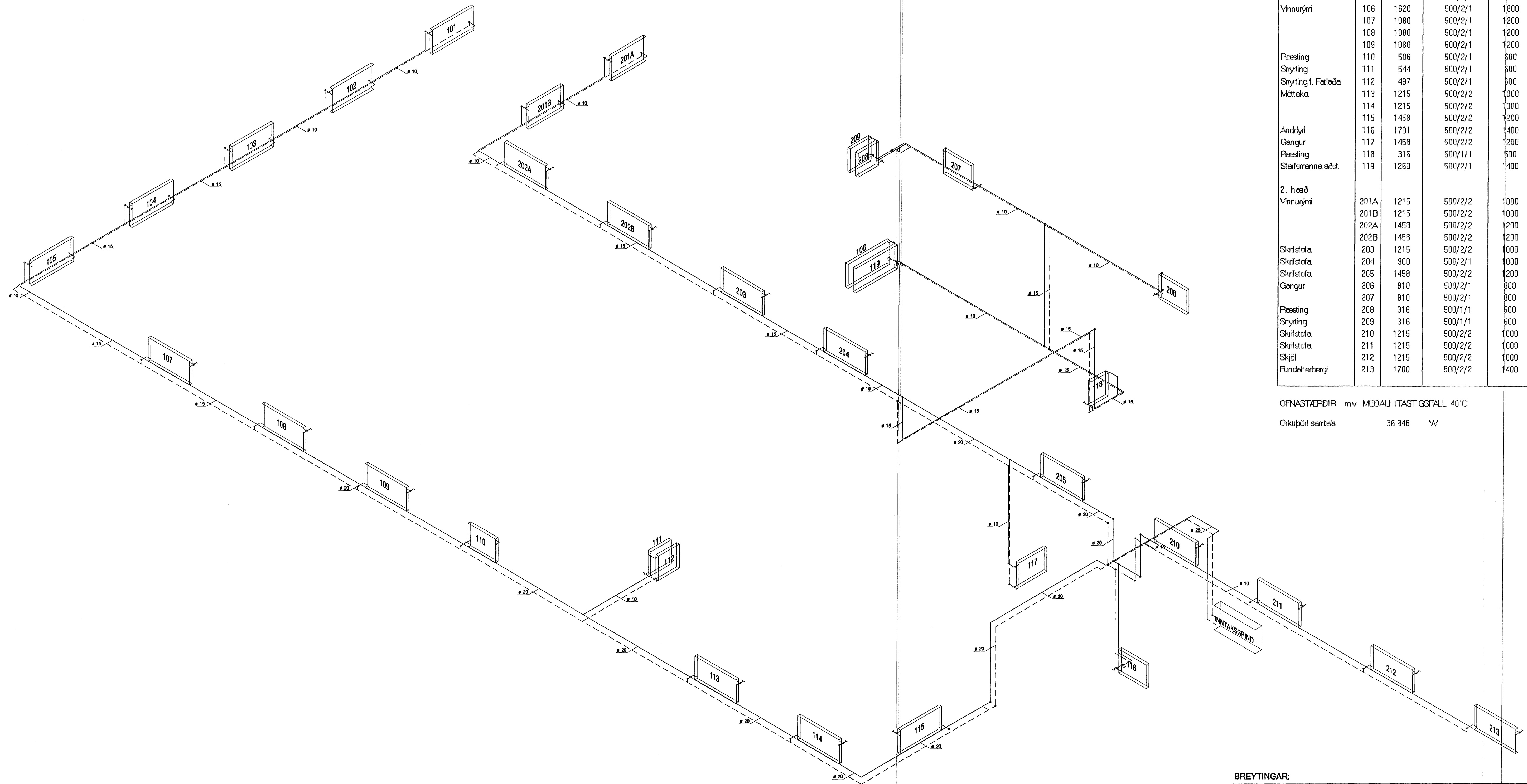
RÚMMYND OFNALAGNA mkv. 1:50
