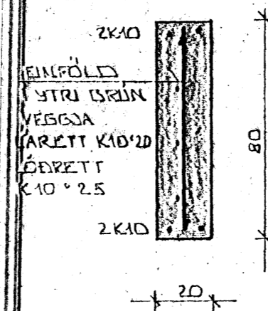
SÚLA S 1.9. 1:20
