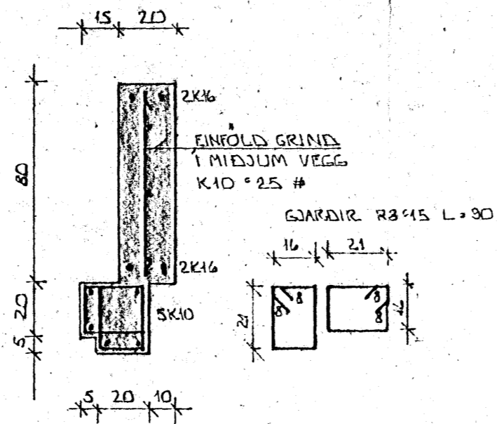
SÚLA S 1.6. 1:20
