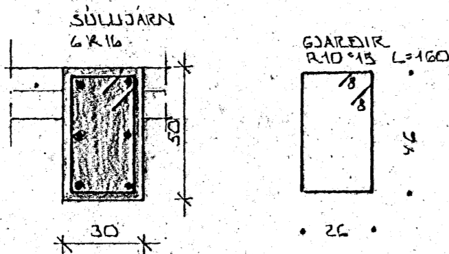
SÚLA S 1.2. 1:20
