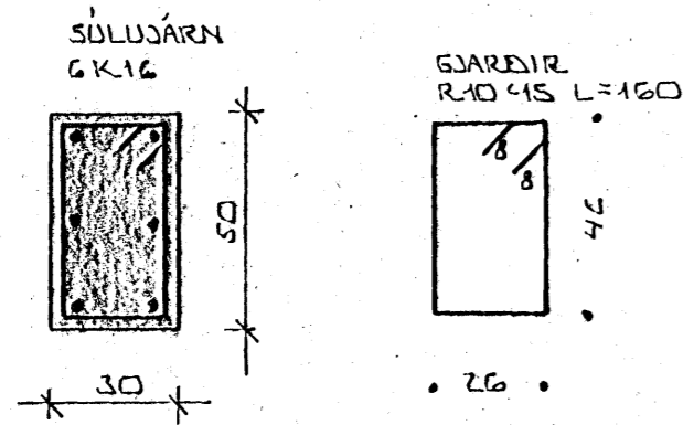
SÚLA S 1.1. 1:20
