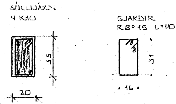
SÚLA S 1.7. 1:20
