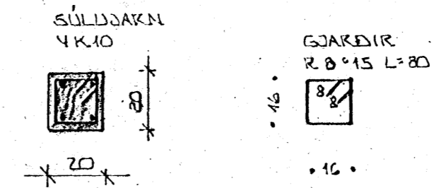
SÚLA S 1.8. 1:20
