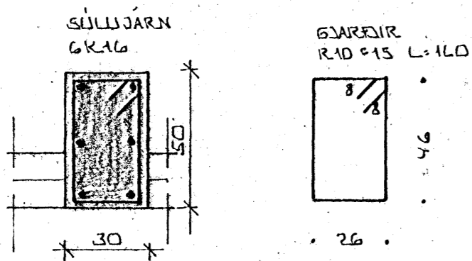
SÚLA S 1.3. 1:20
