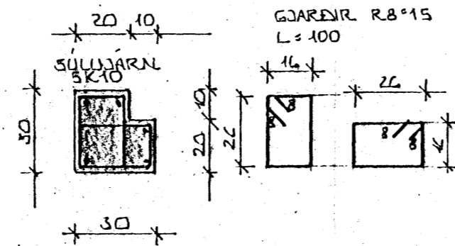
SÚLA S 1.4. 1:20
