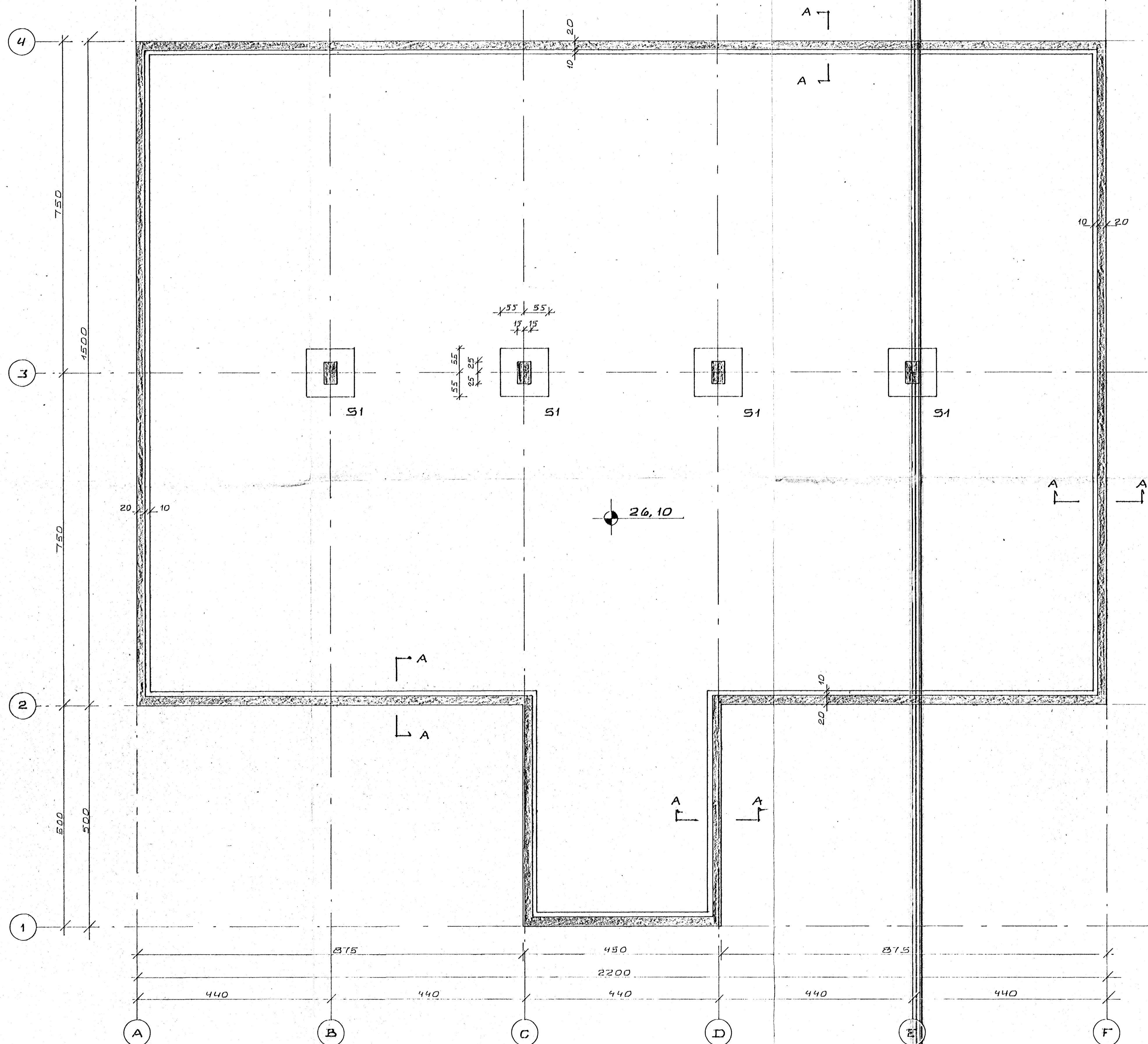
GRUNNMYND 1:50
