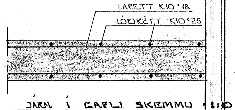
JARN I GARLI SKEMMU 1:10
