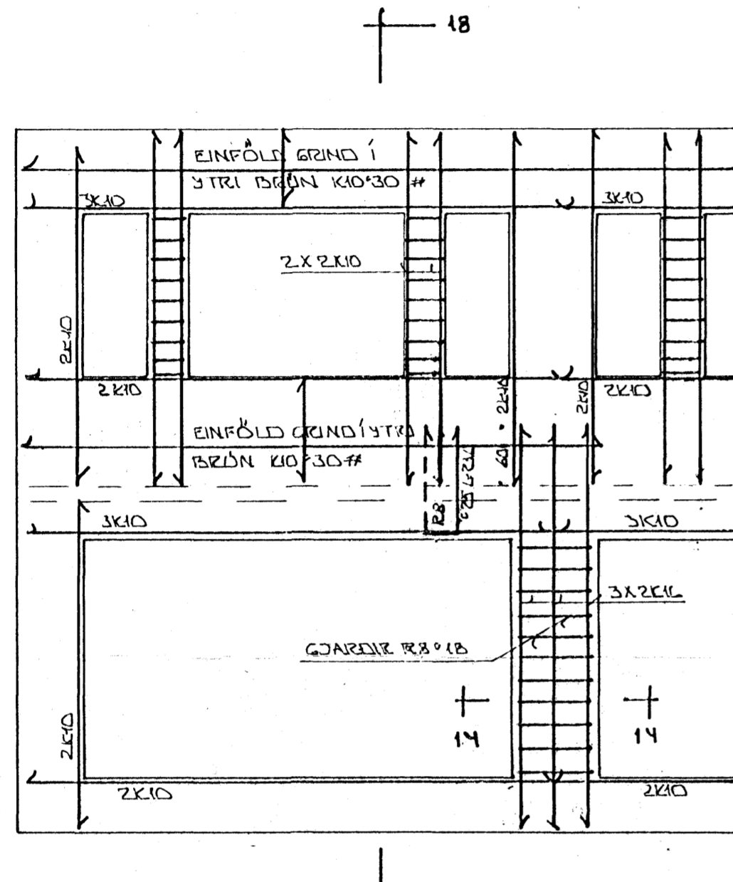
KENNISNIÐ Í ÚTVEGG \sim 1:50
