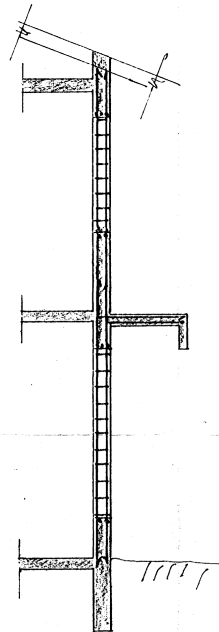
SNÍÐ 18-18 \sim 1:50
