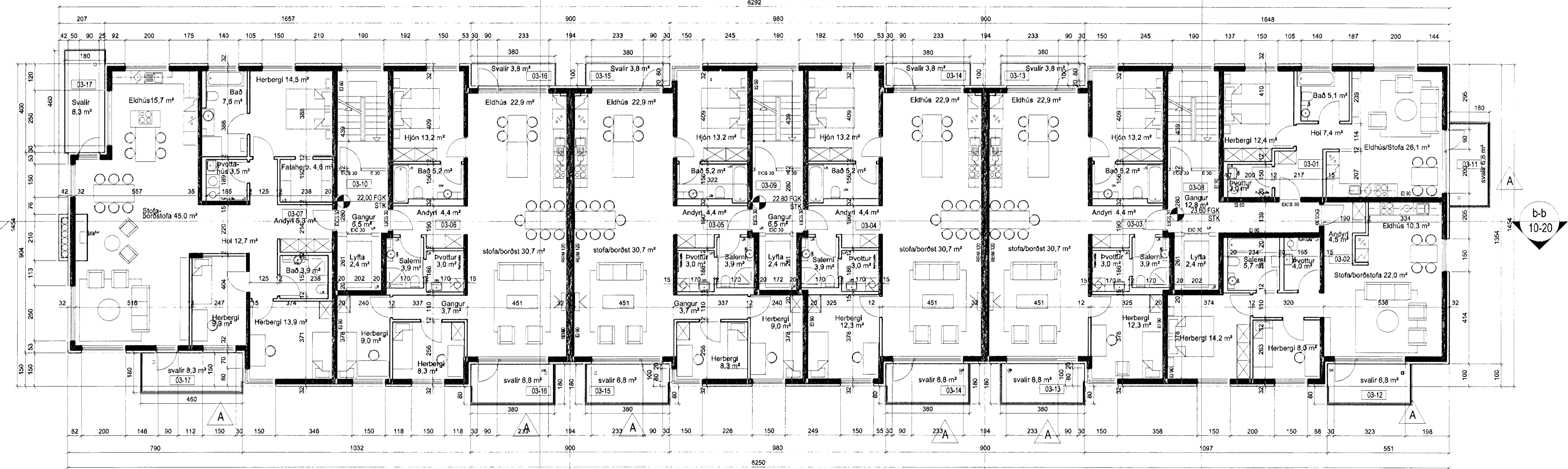
GRUNNMYND 3. HÆÐ 1:100
