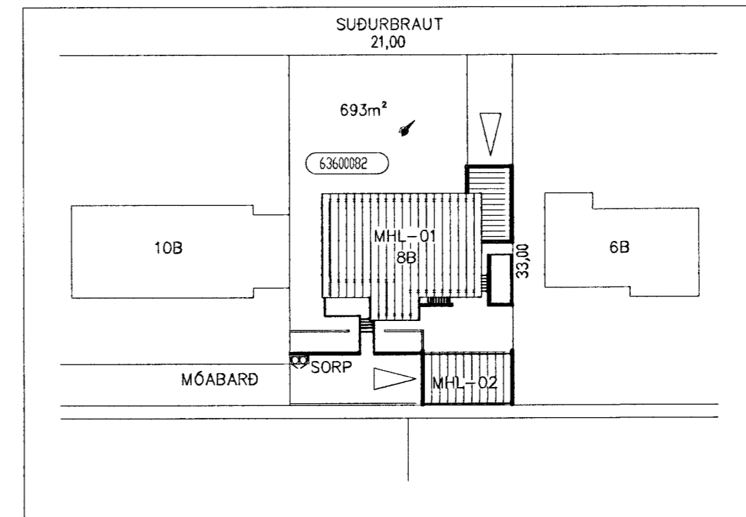
AFSTÖÐUMYND 1:500
