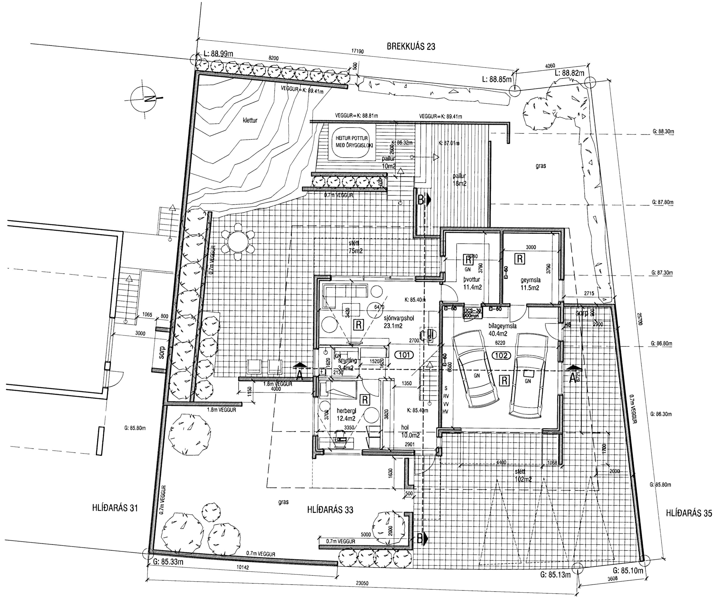
Grunnmynd mkv. 1:100
