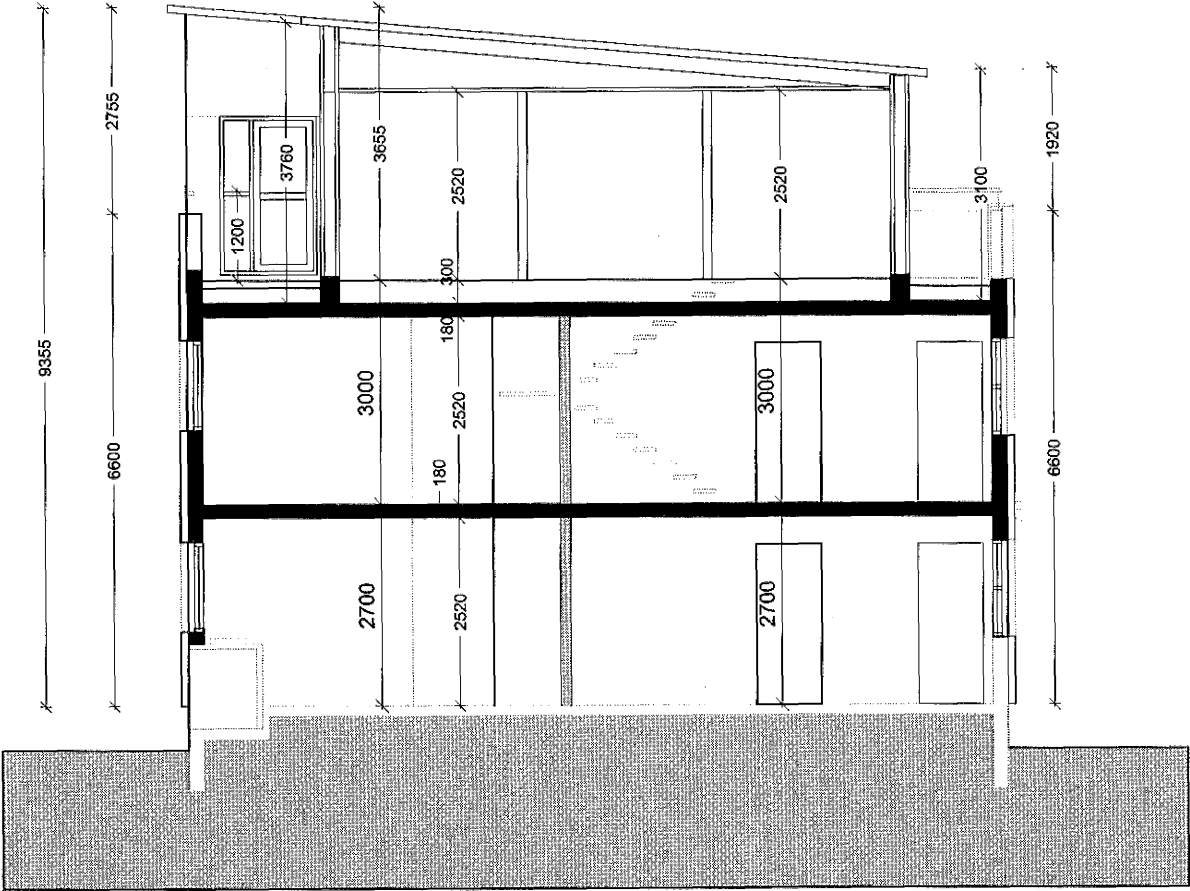
Snið A-A
