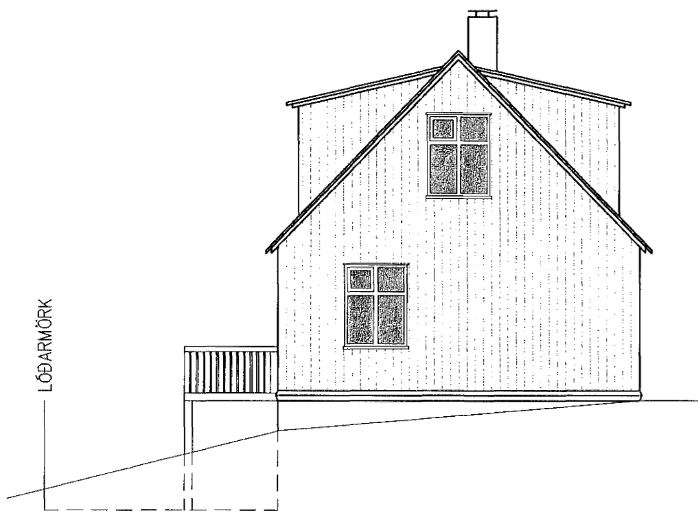
SUÐUR MKV. 1:100
