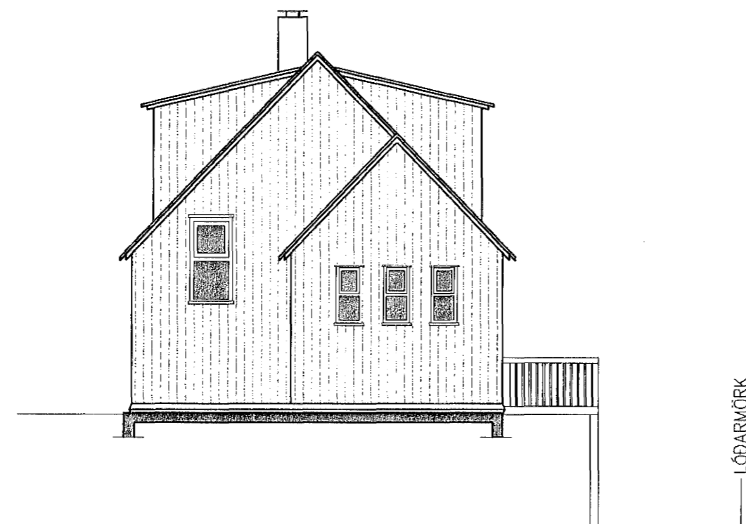
NORÐUR MKV. 1:100
