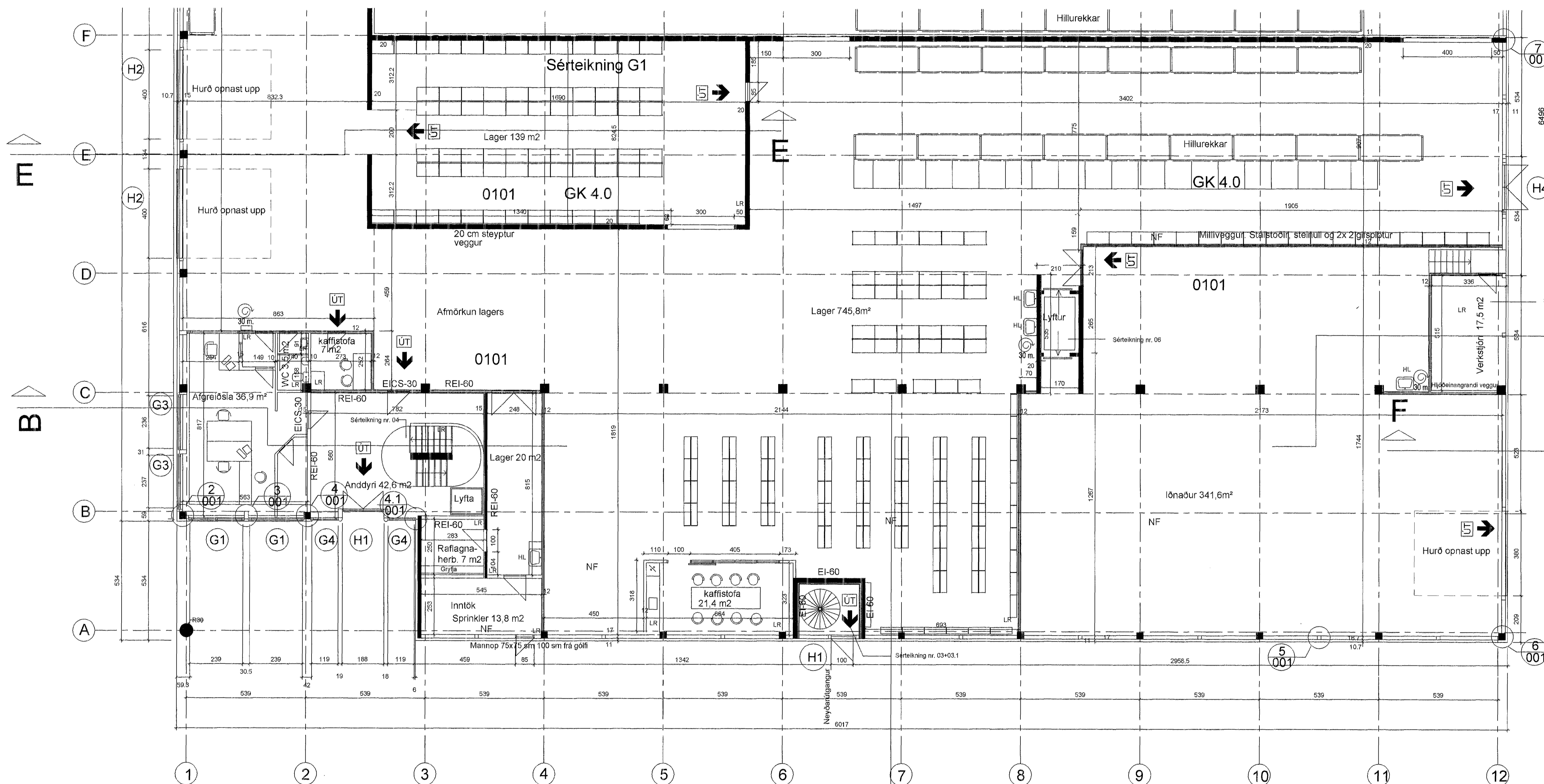
Grunnmynd 1. hæðar, hluti 2
