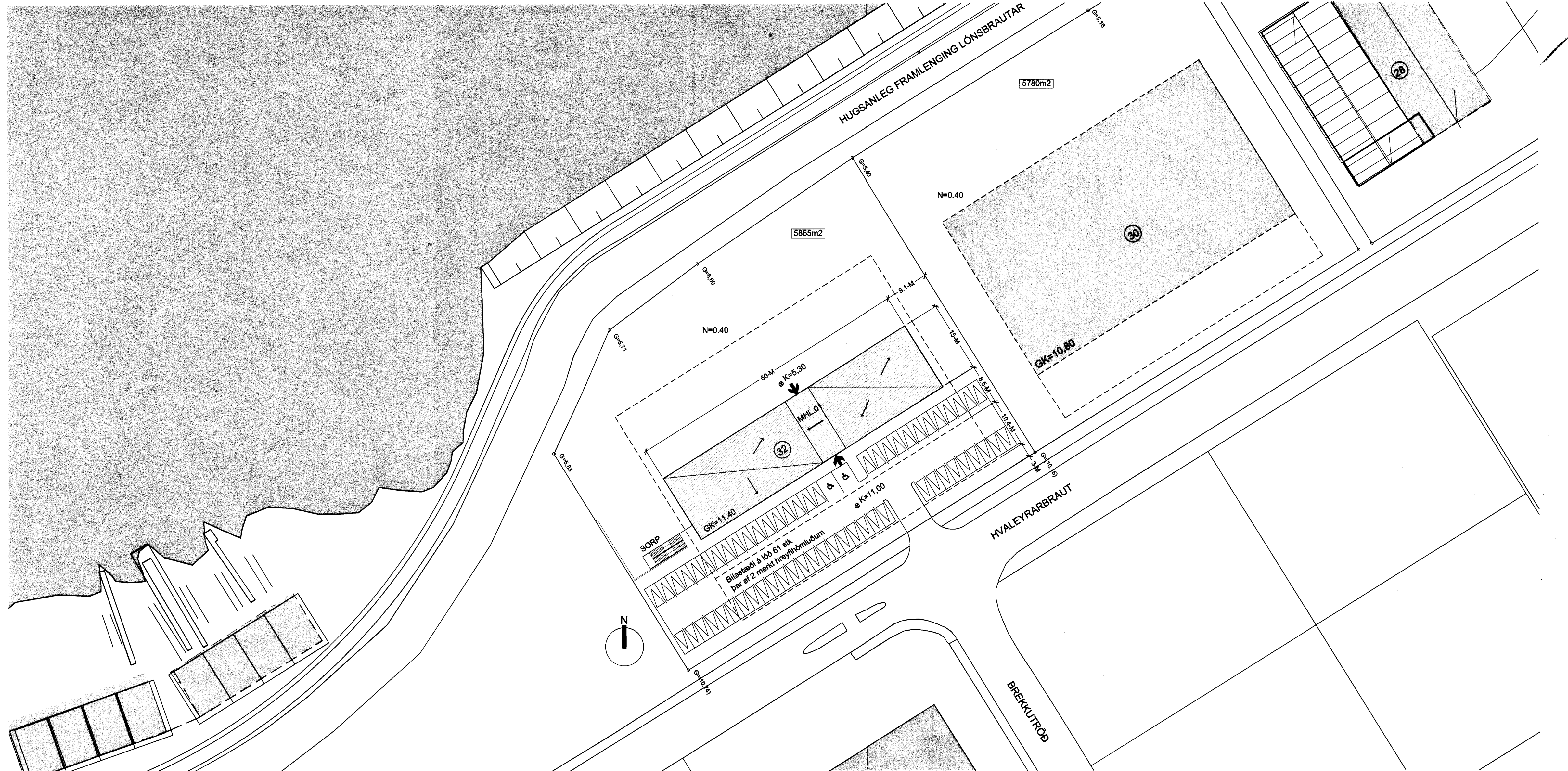
AFSTÖÐUMYND MKV 1:500
