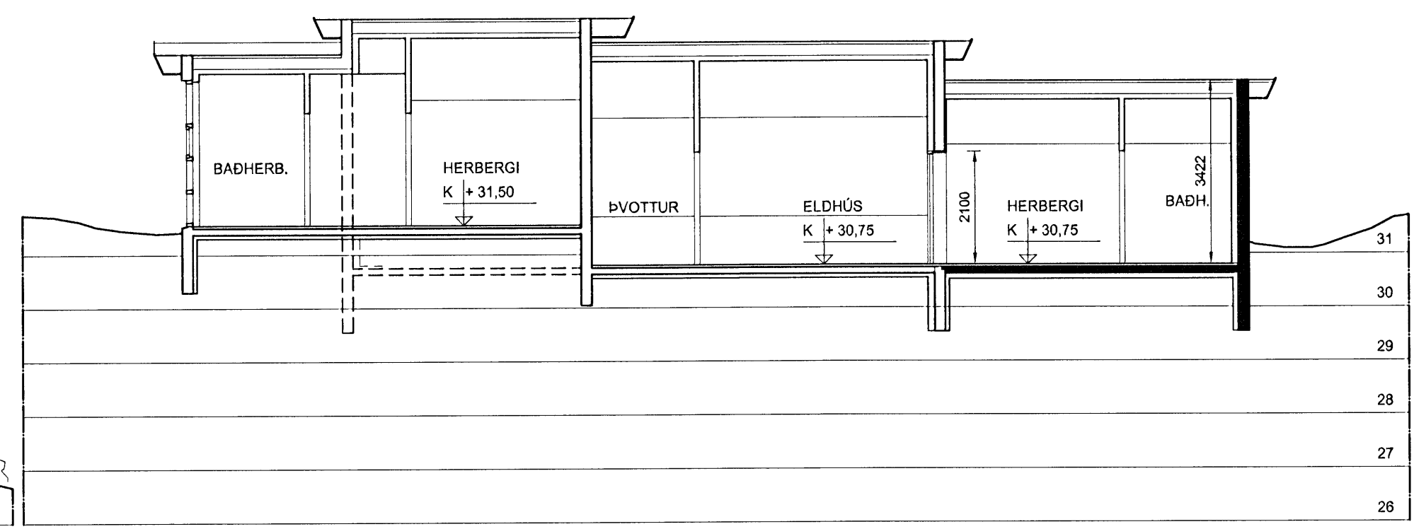
SNEIÐING D - D
