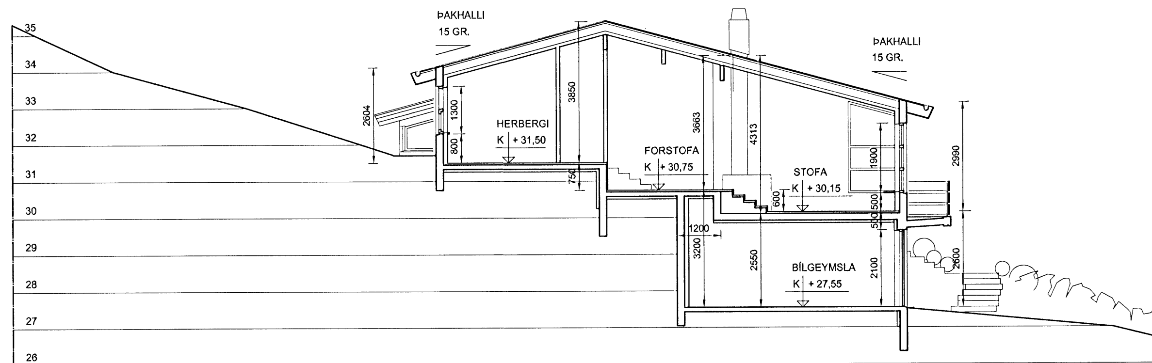
SNEIÐING B - B
