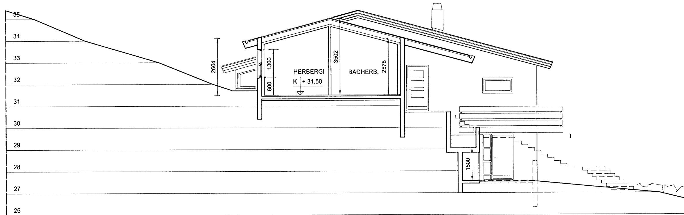
SNEIÐING A - A
