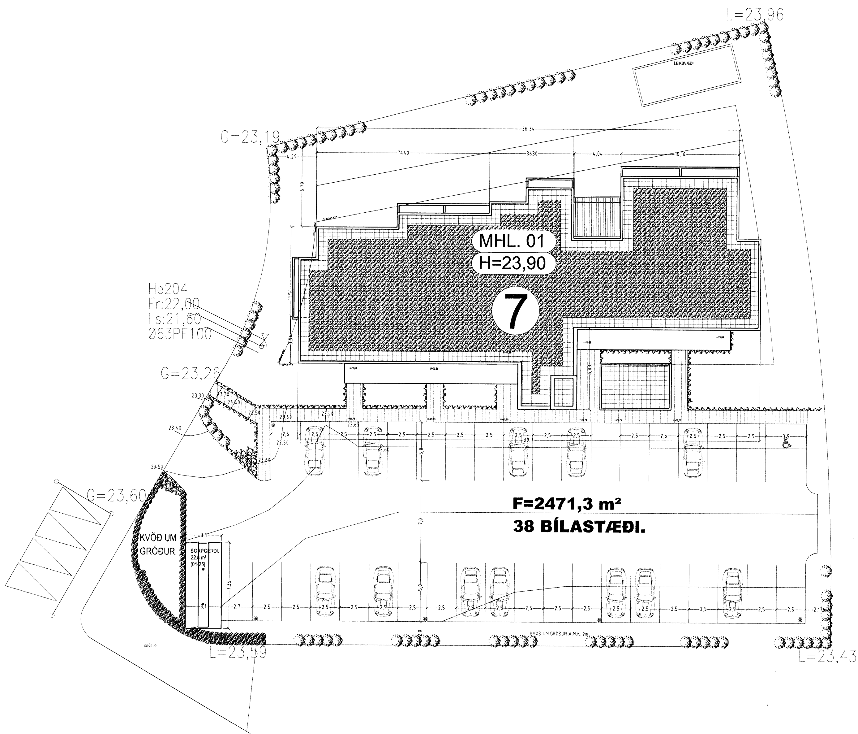
LÓÐARMYND MKV. 1:200.
