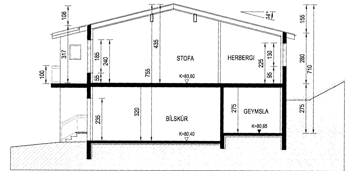
SNID A-A
