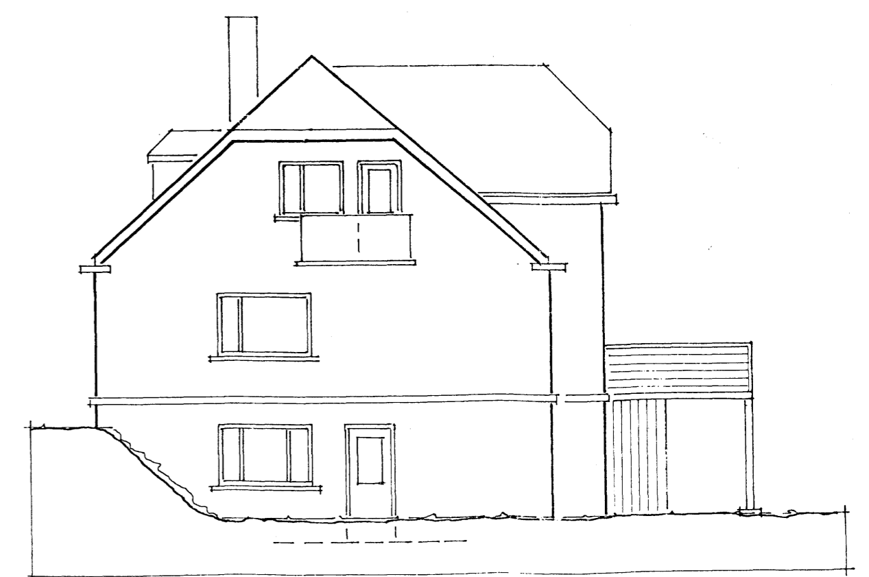
ÚTLIT NORÐVESTUR 1:100
