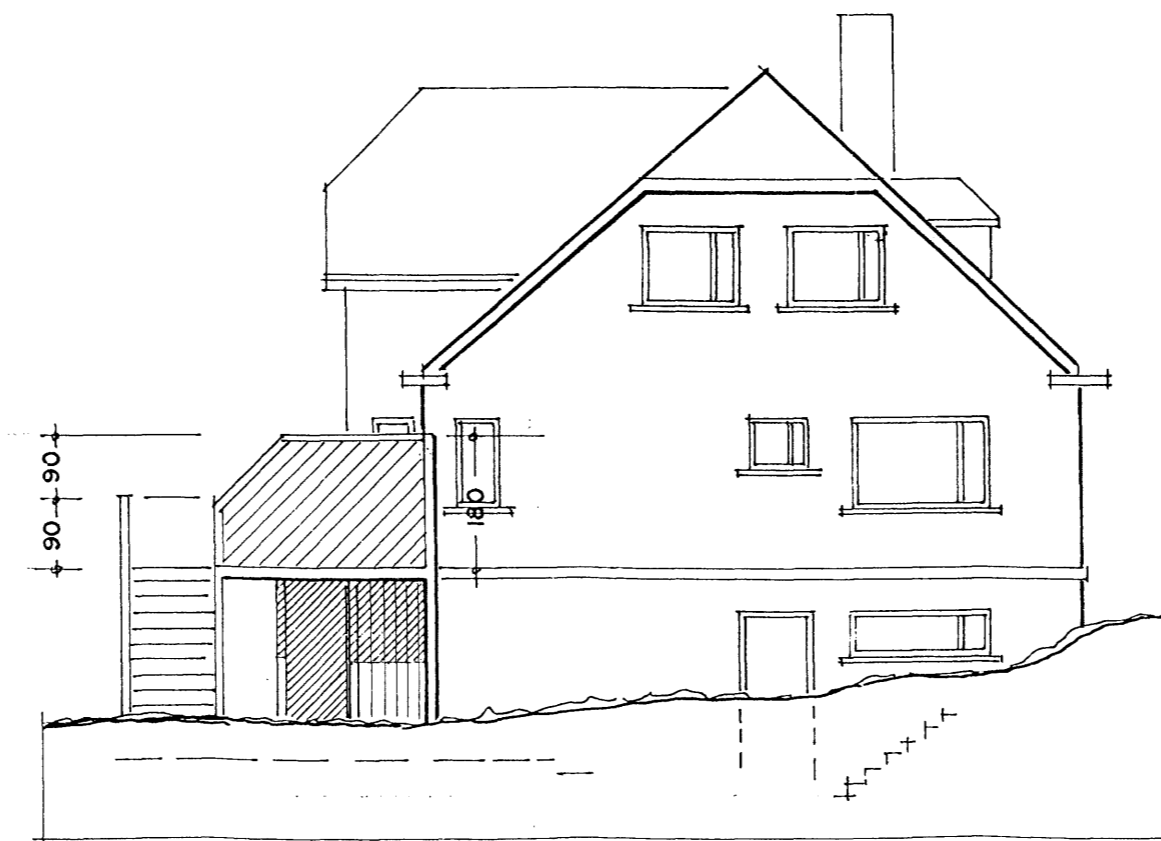
ÚTLIT SUÐAUSTUR 1:100
