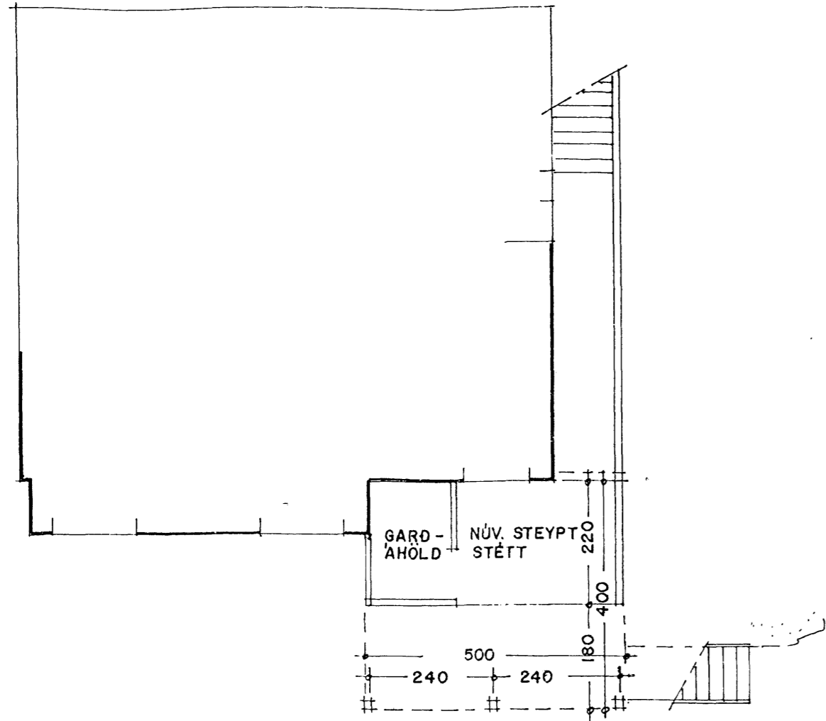
GRUNNMYND KJALLARA 1:100
