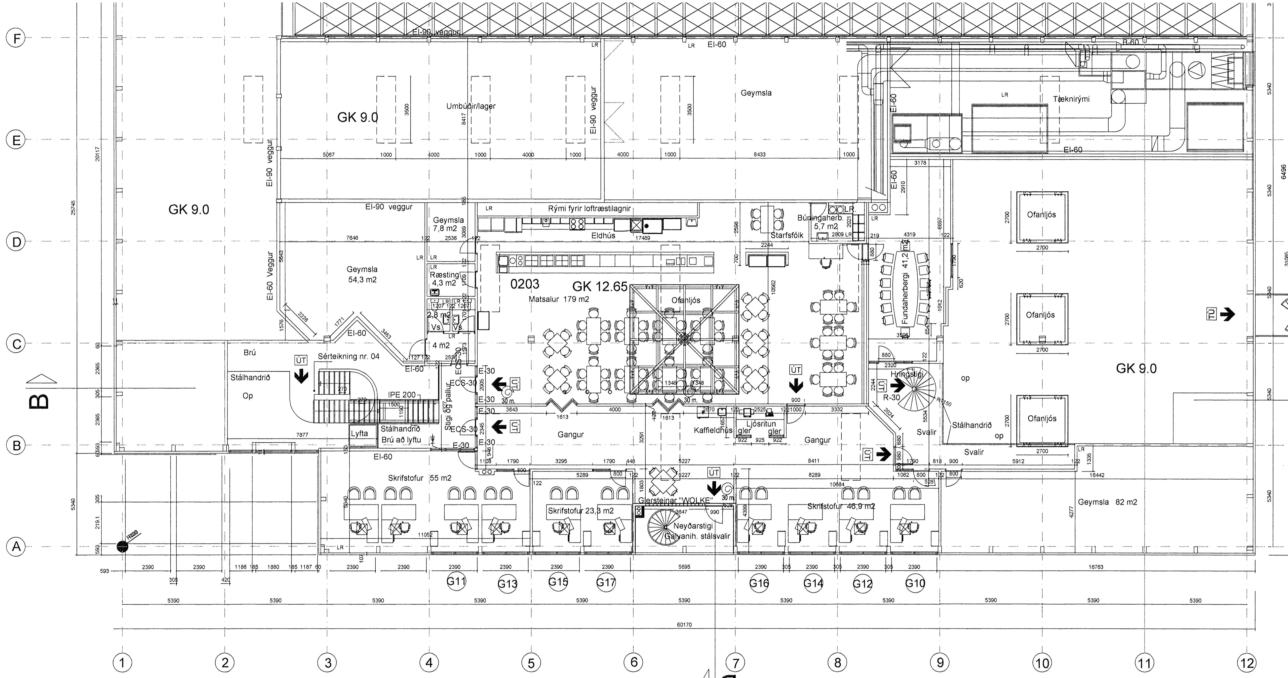
Grunnmynd 3. hæðar
