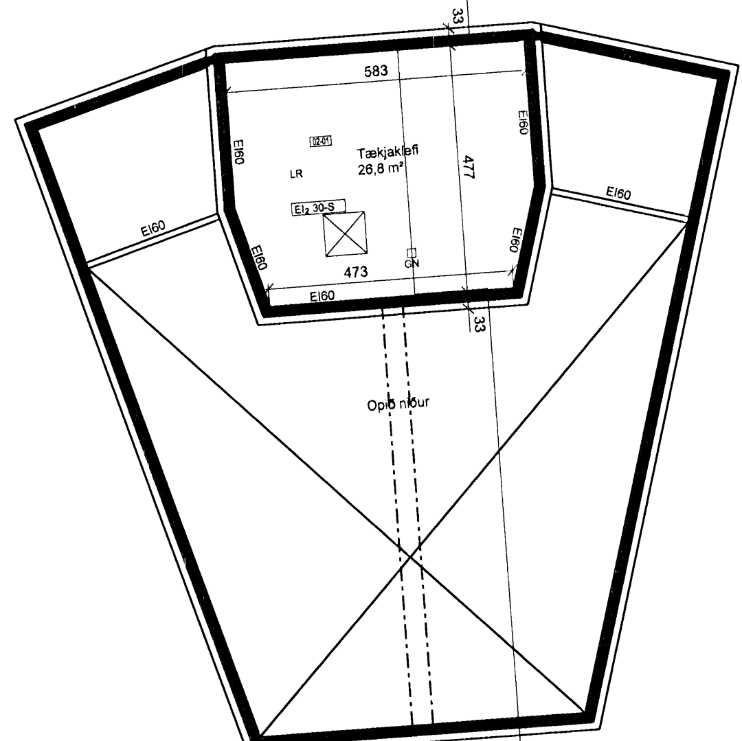
GRUNNMYND 1:100 2. hæð
