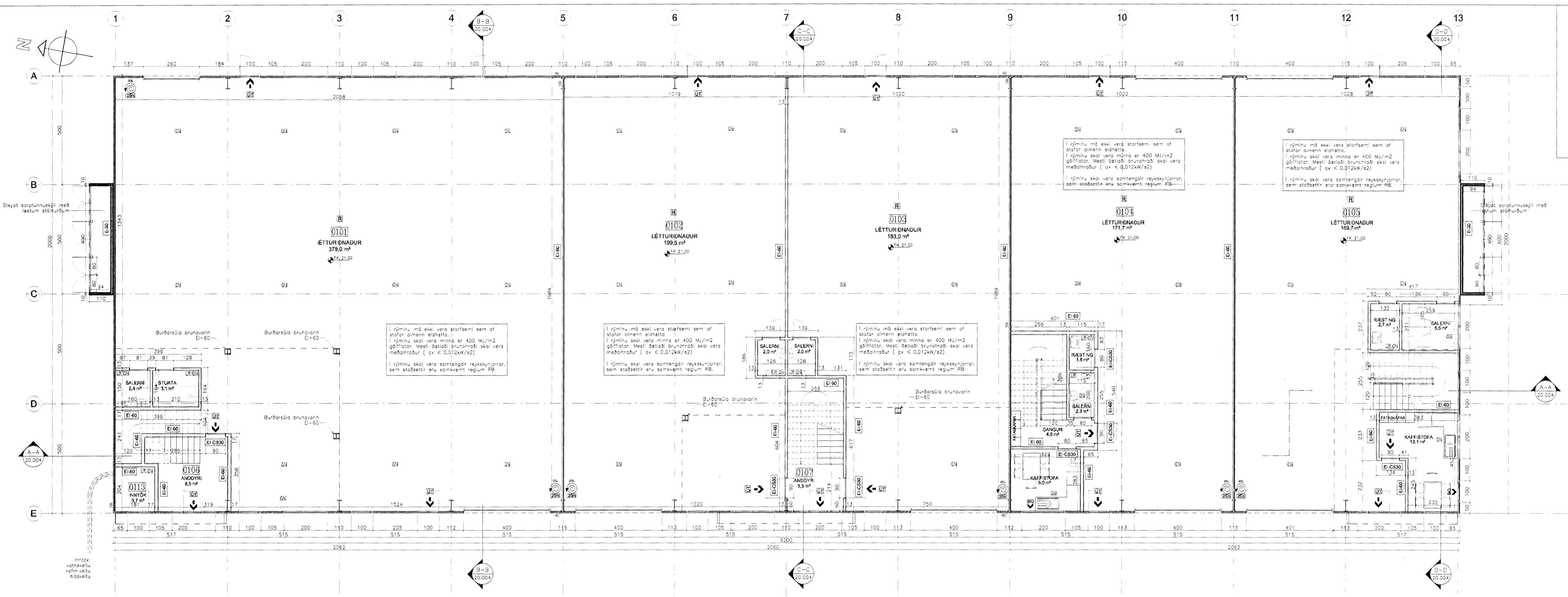
GRUNNMYND 1.HÆÐ 1:100
