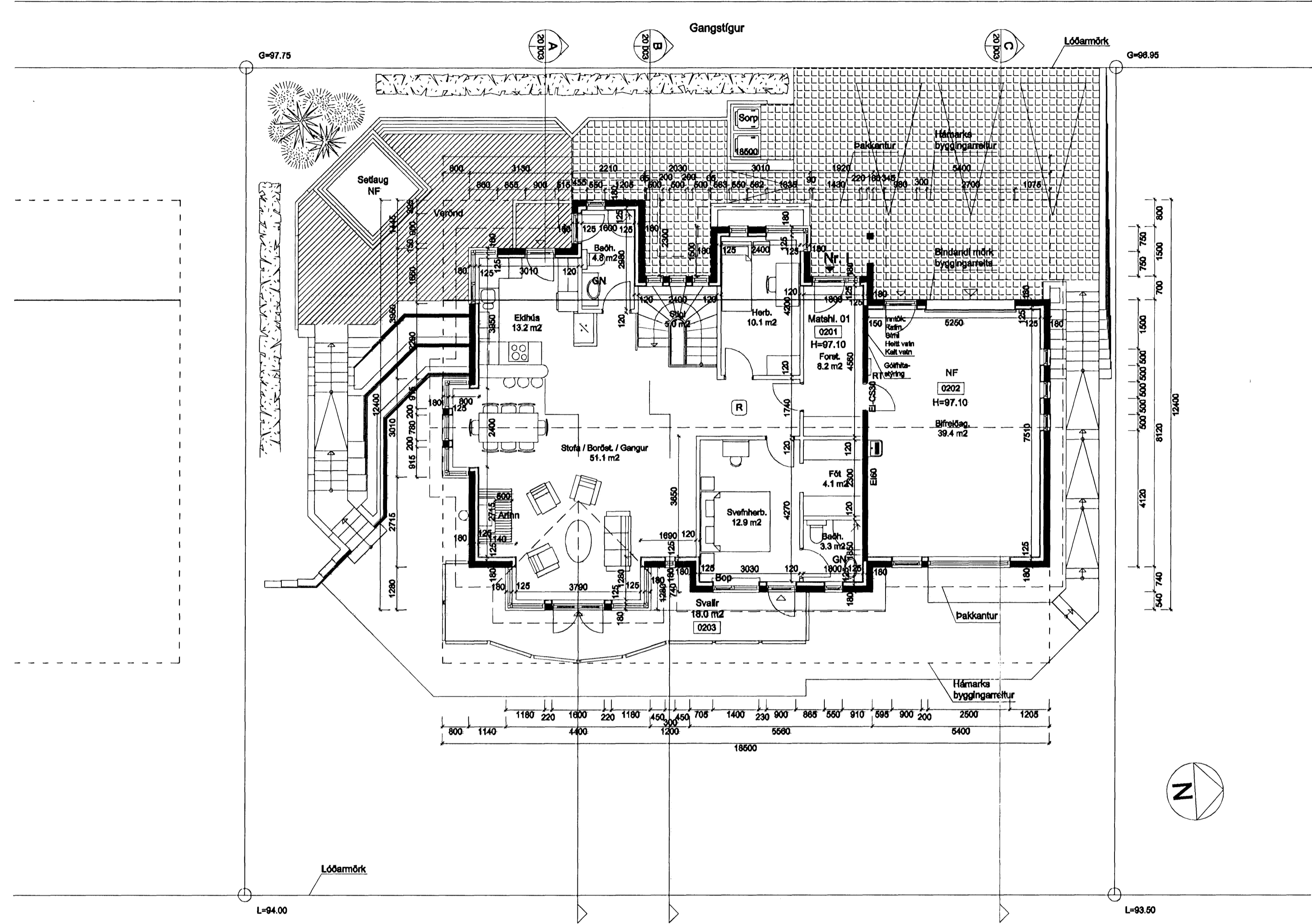
Grunnmynd 2. hæðar
