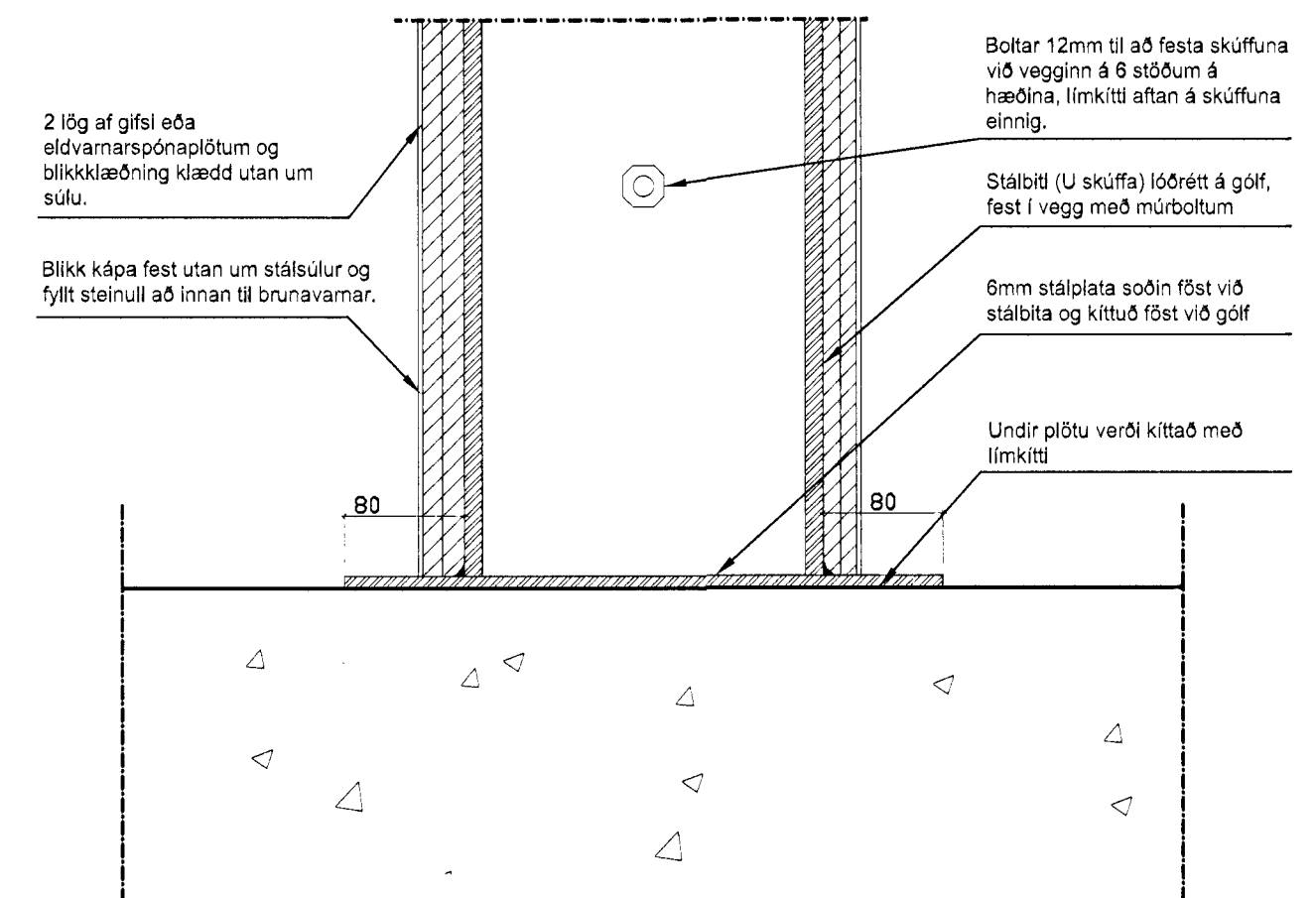
4 Lóðrétt og lárétt deili 200 Frágangur við gólf
