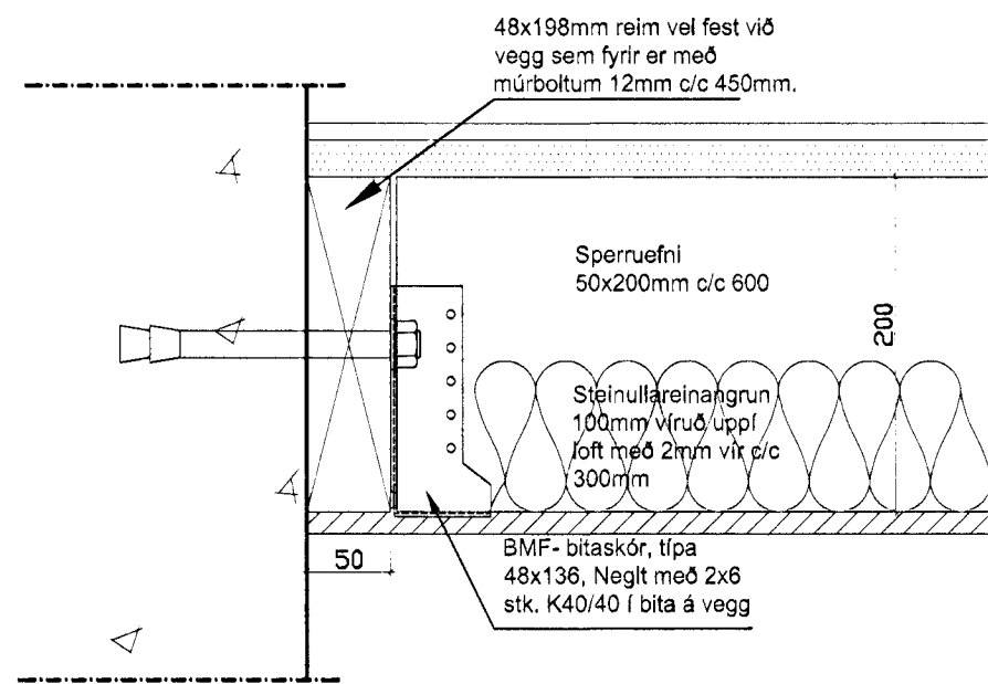
1 Lóðrétt deili 200 Frágangur við milliloft
