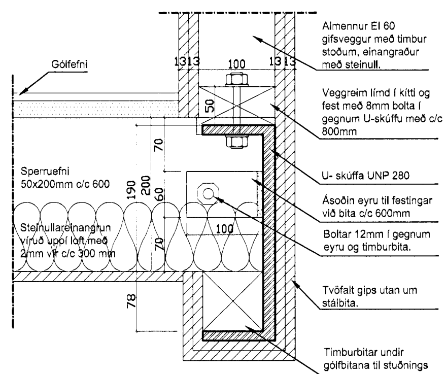
3 Lóðrétt deili 200 Frágangur við milliloft
