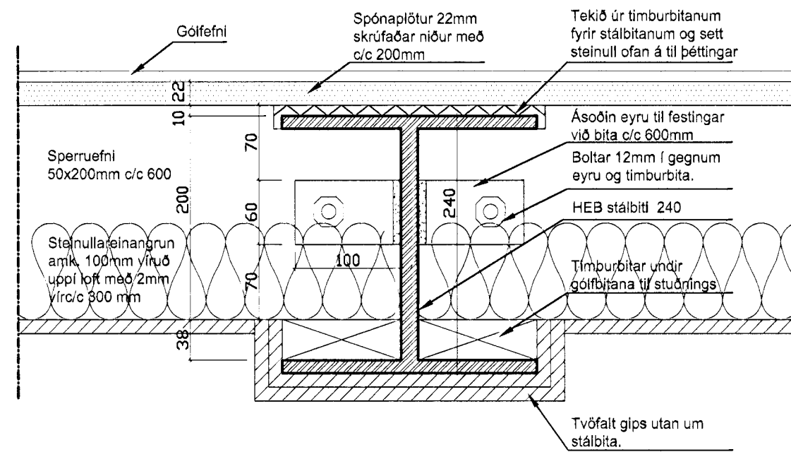
2 Lóðrétt deili 200 Frágangur við milliloft
