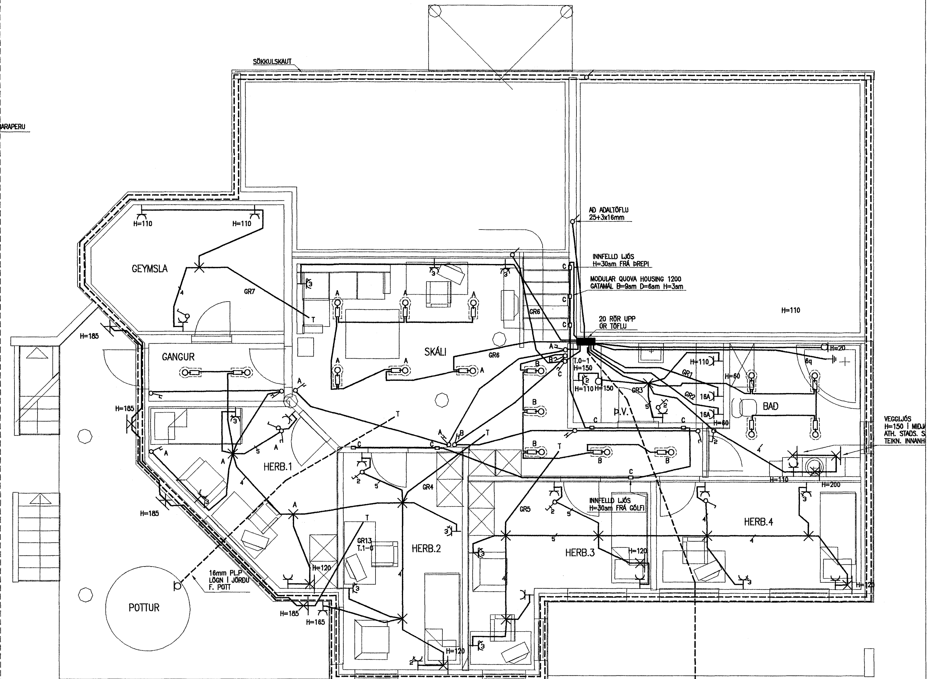
NEDRI HÆÐ
