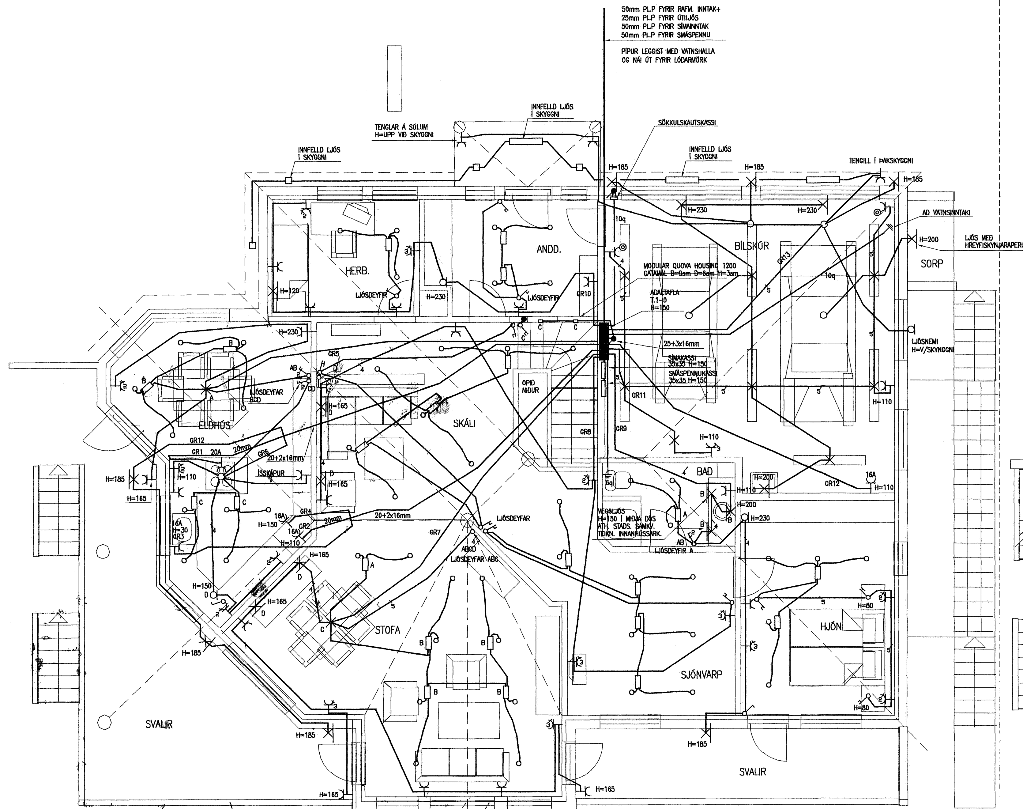
EFRI HÆÐ
