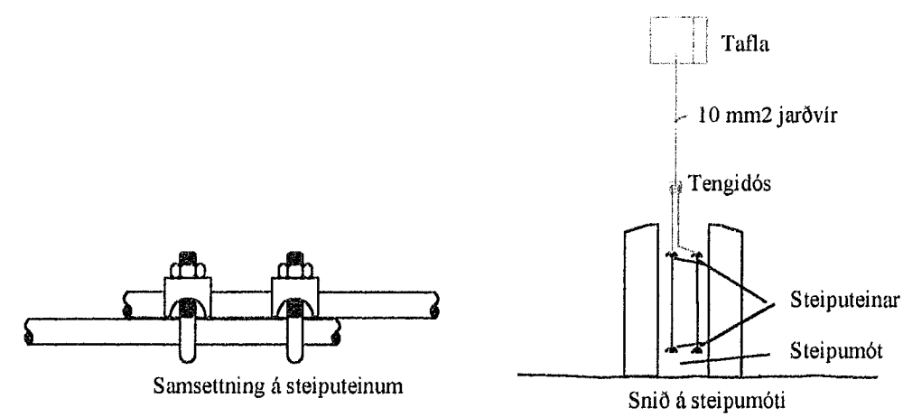
Tenging sökkulskauts Taka skal upp tvo teina og tengja saman í tengibox undir töflu
