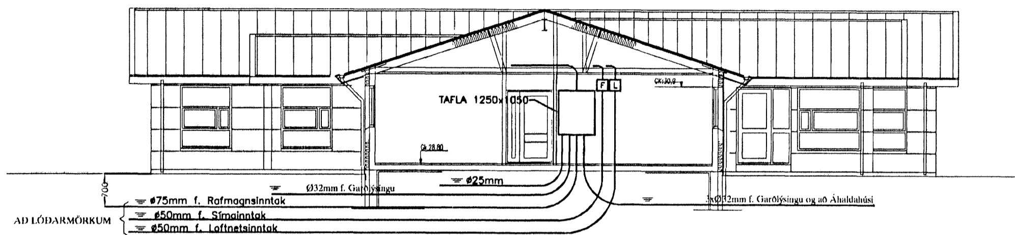
SNÍÐ A-A Í INNTAK M 1:100
