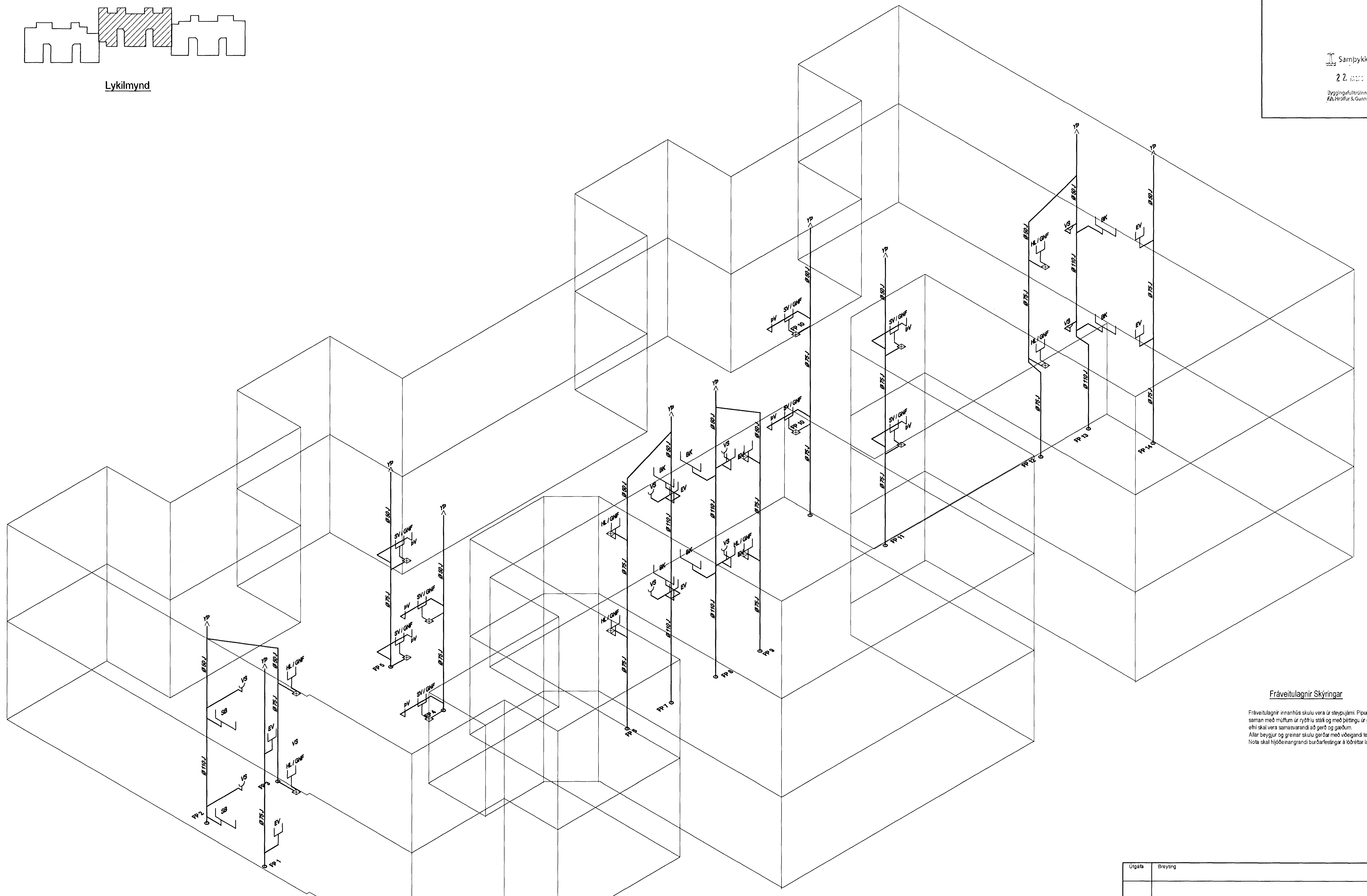
Fráveitulagnir, Rúmmynd, 1:50
