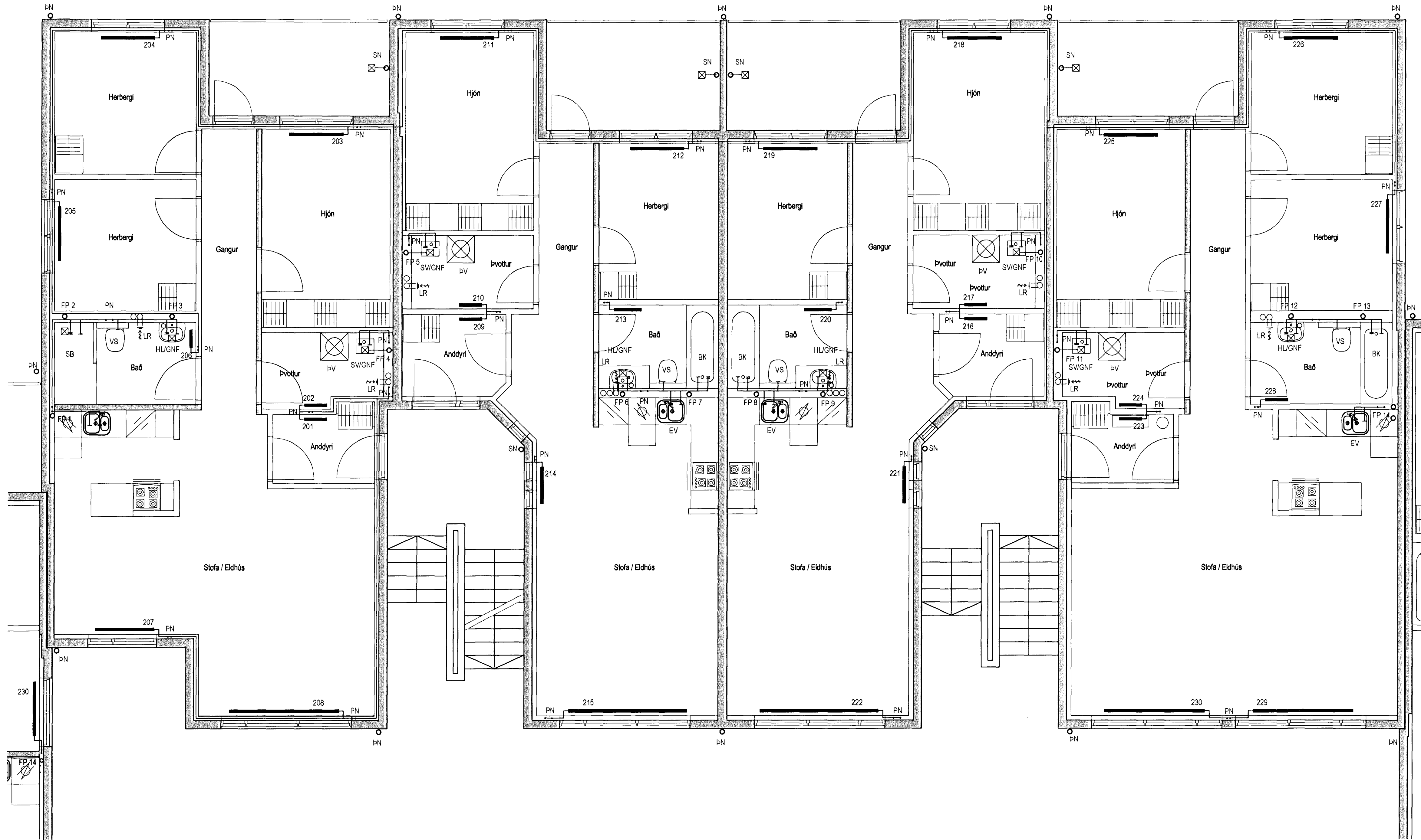
Lagnir 2. hæð, Grunnmynd 1:50
