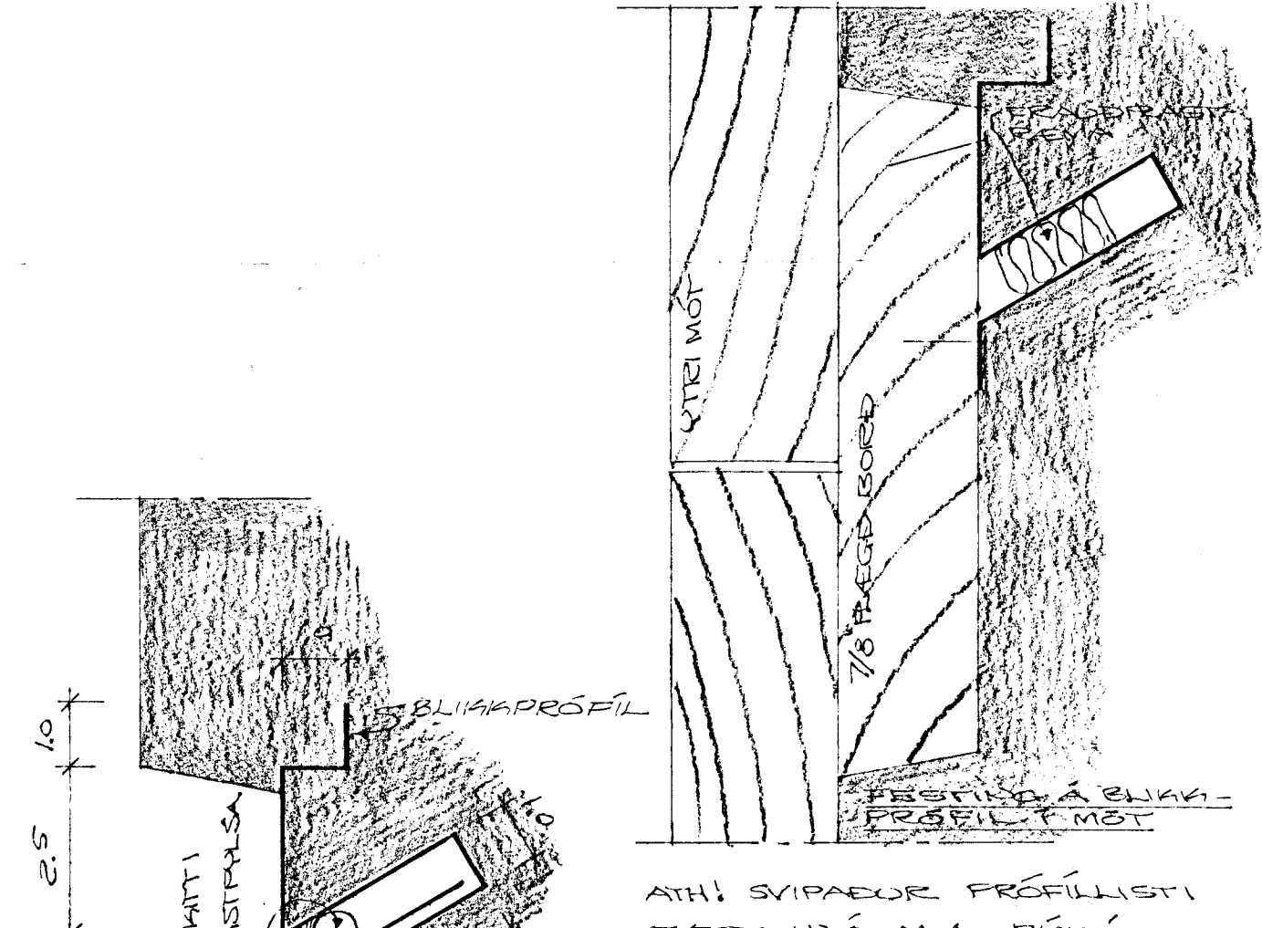
SKURÐUR D, M=1:20
