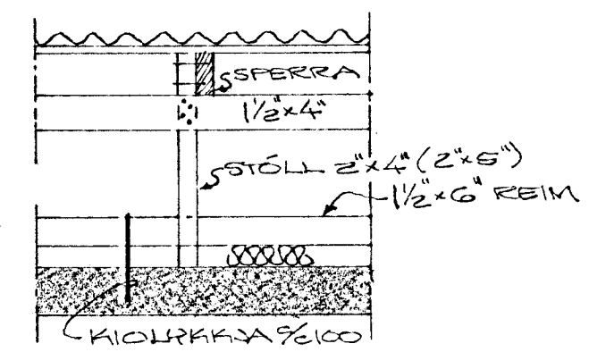
SKURÐUR B, M=1:20
