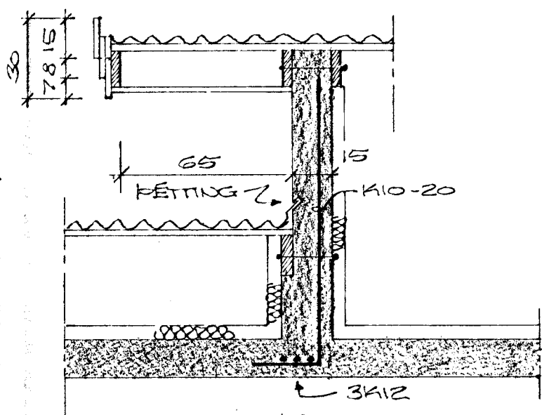
GRUNNDRAG, M=1:50
