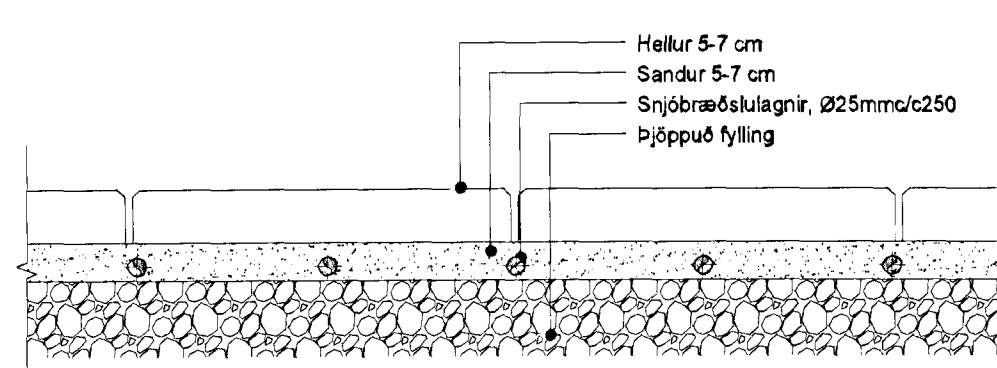
KENNISNIÐ SNJÓBRÆÐSLU Í HELLUR 1:10
