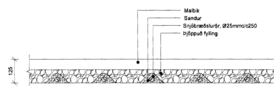
KENNISNIÐ SNJÓBRÆÐSLU Í MALBIK 1:10
