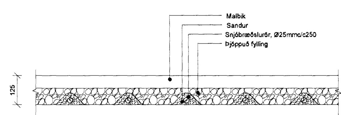
KENNISNIÐ SNJÓBRÆÐSLU Í MALBIK 1:10
