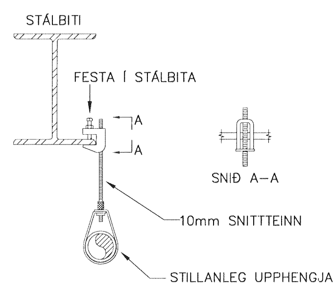
UPPHENGJA Í STÁLBITA S.061127/agnir/110904N-103
