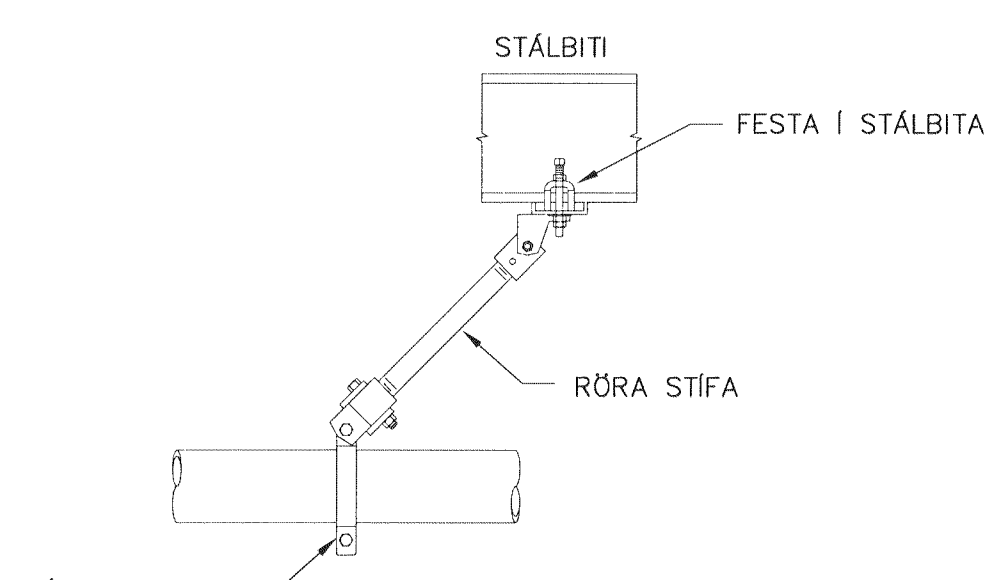
JARÐSKJÁLFTASTÍFA (Í STEFNU RÖRS)
