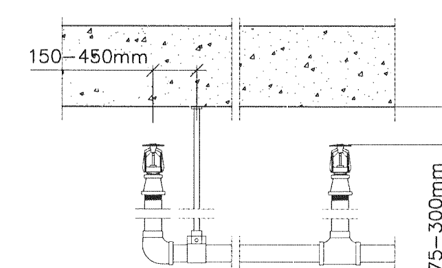
UPPVÍSANDI ÚÐASTÚTAR (Ú1)
