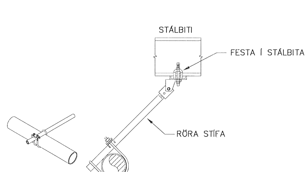
JARÐSKJÁLFTASTÍFA (ÞVERSTÍFA)
