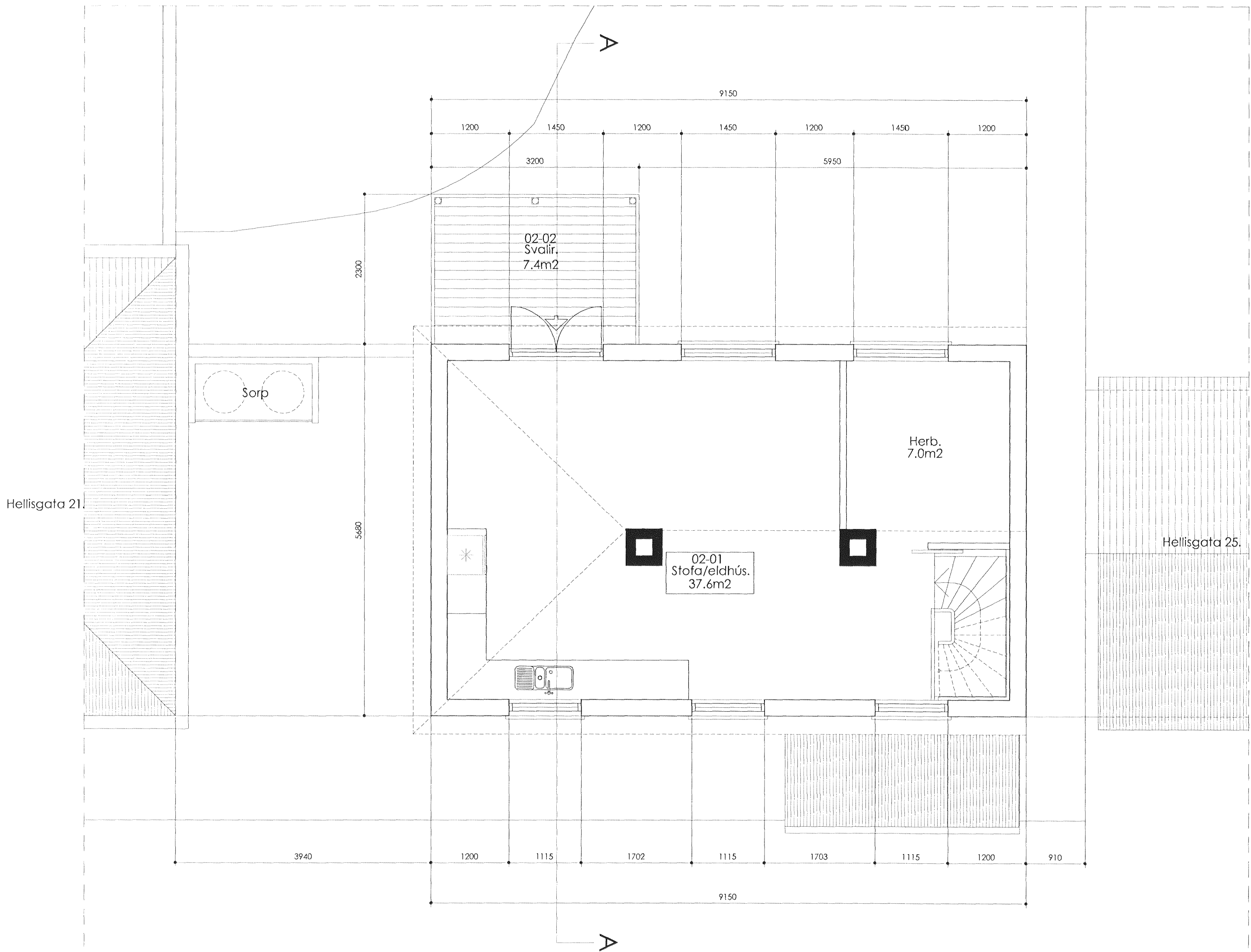
Grunnmynd 2. hæðar.
