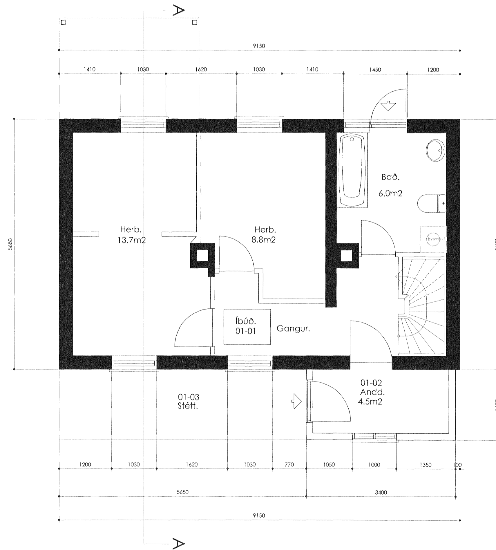
Grunnmynd 1. hæðar.
