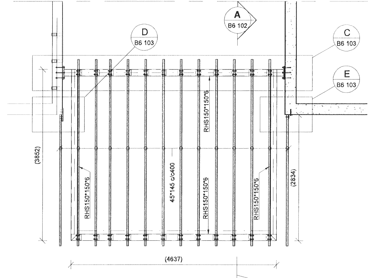
Vindfang II, Ofanmynd þaks 1:50
