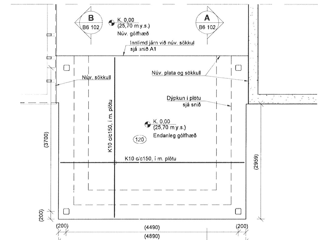
Vindfang II, Grunnmynd undirstaða og plötu 1:50
