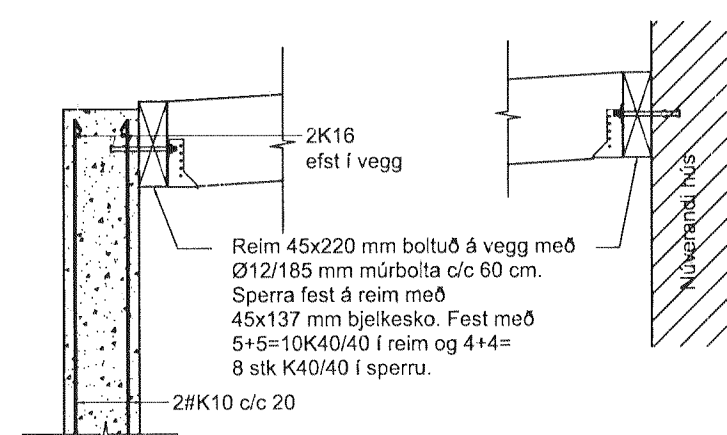
1.1 Sérmynd 1.1. 1:20.
