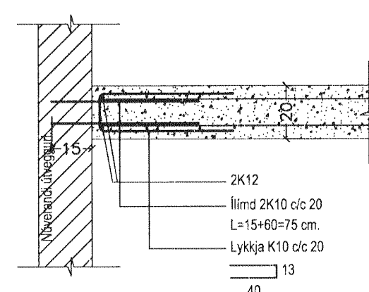
1.2 Sérmynd 1.2. 1:20.
