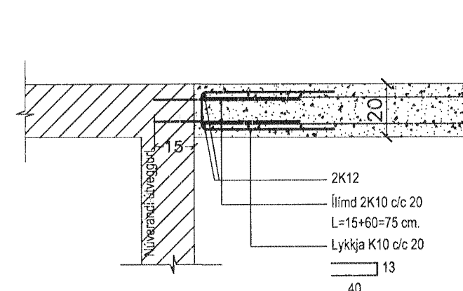
1.3 Sérmynd 1.3. 1:20.
