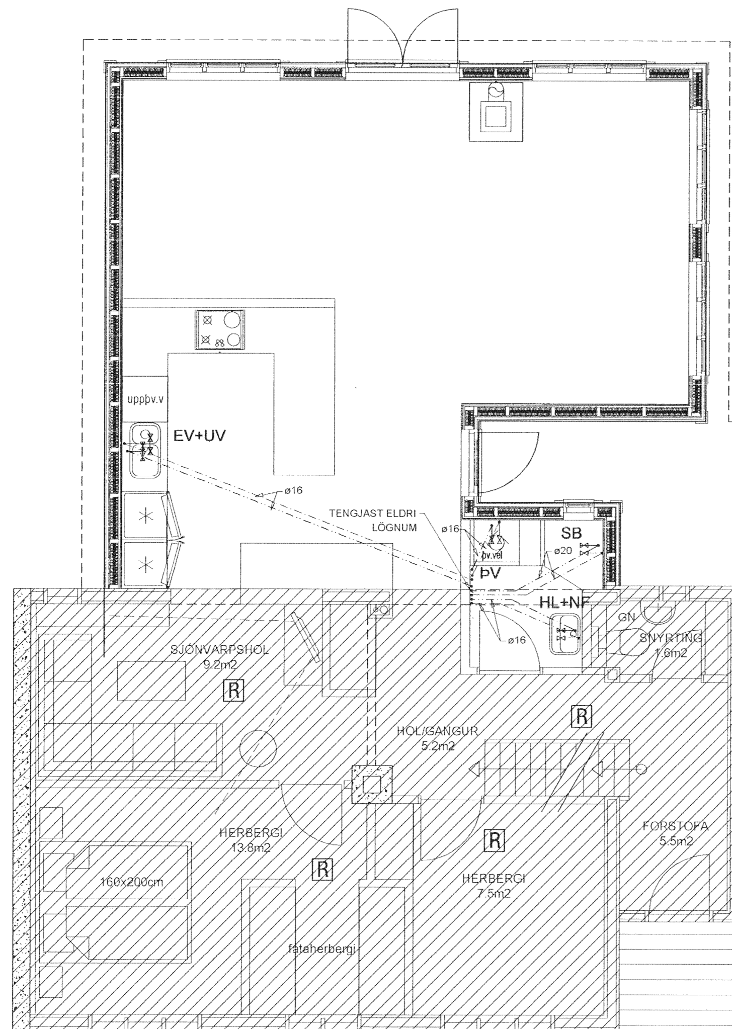
GRUNNMYND NEYSLUVATNSLAGNA, 1:50
