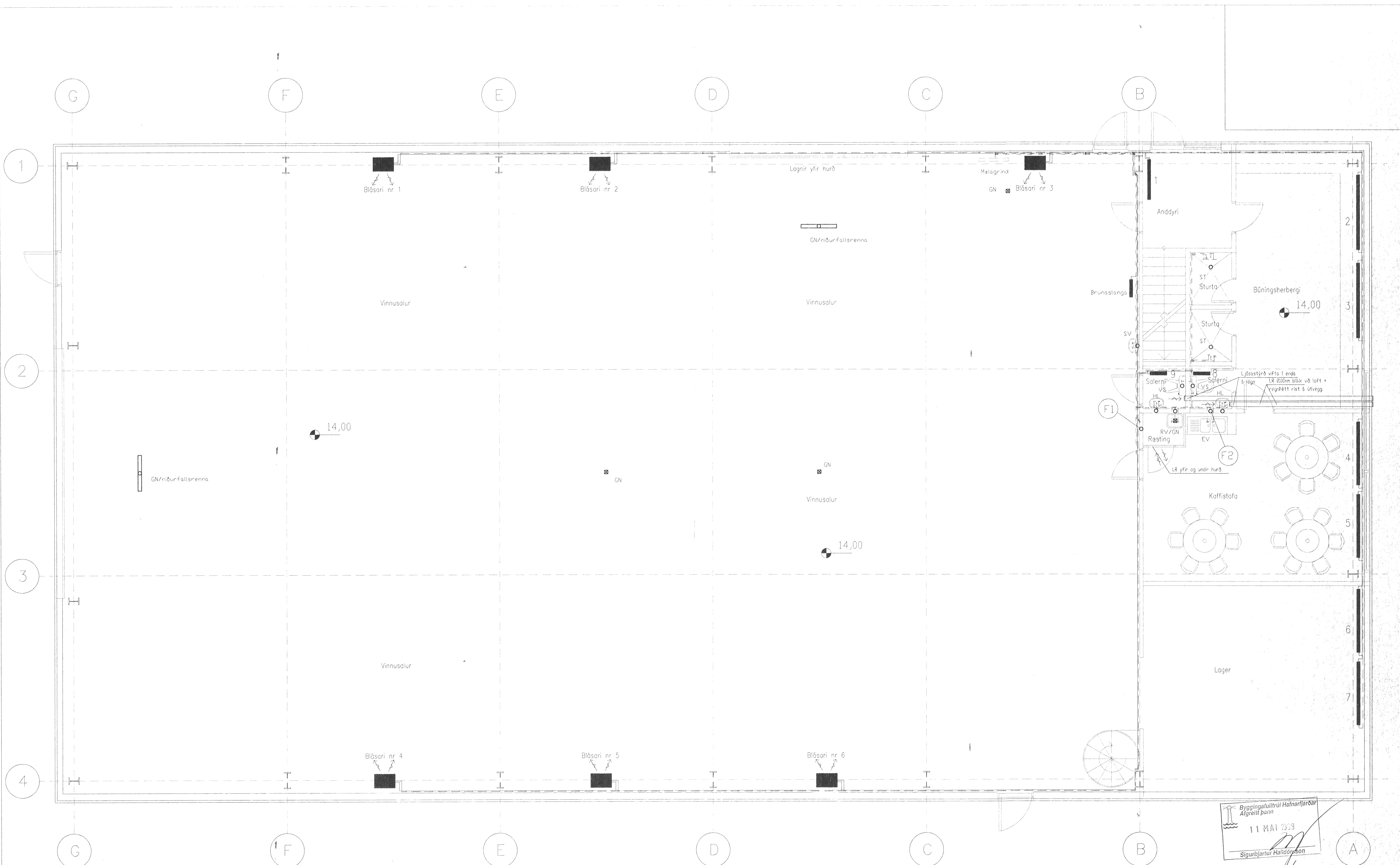
Grunnmynd Jarðhæðar 1:50
