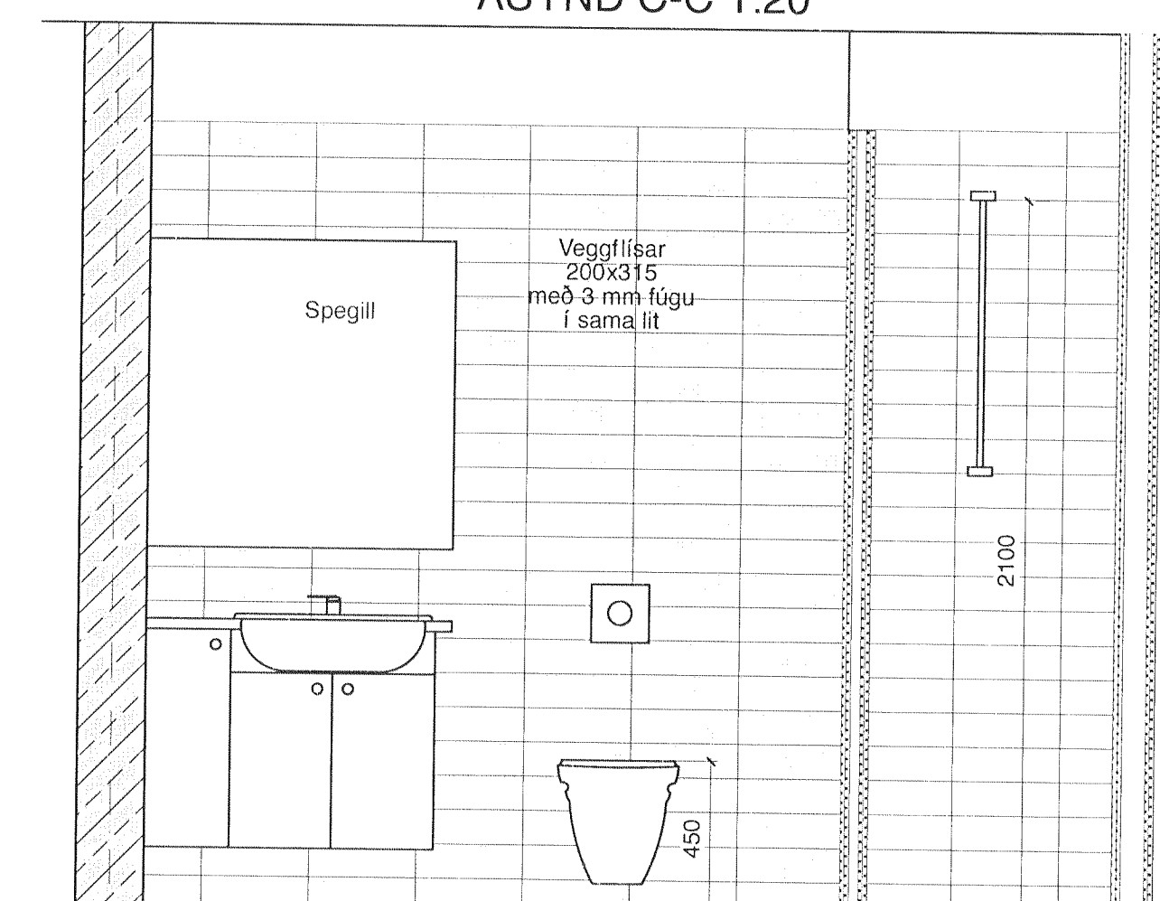
ÁSÝND A-A 1:20
