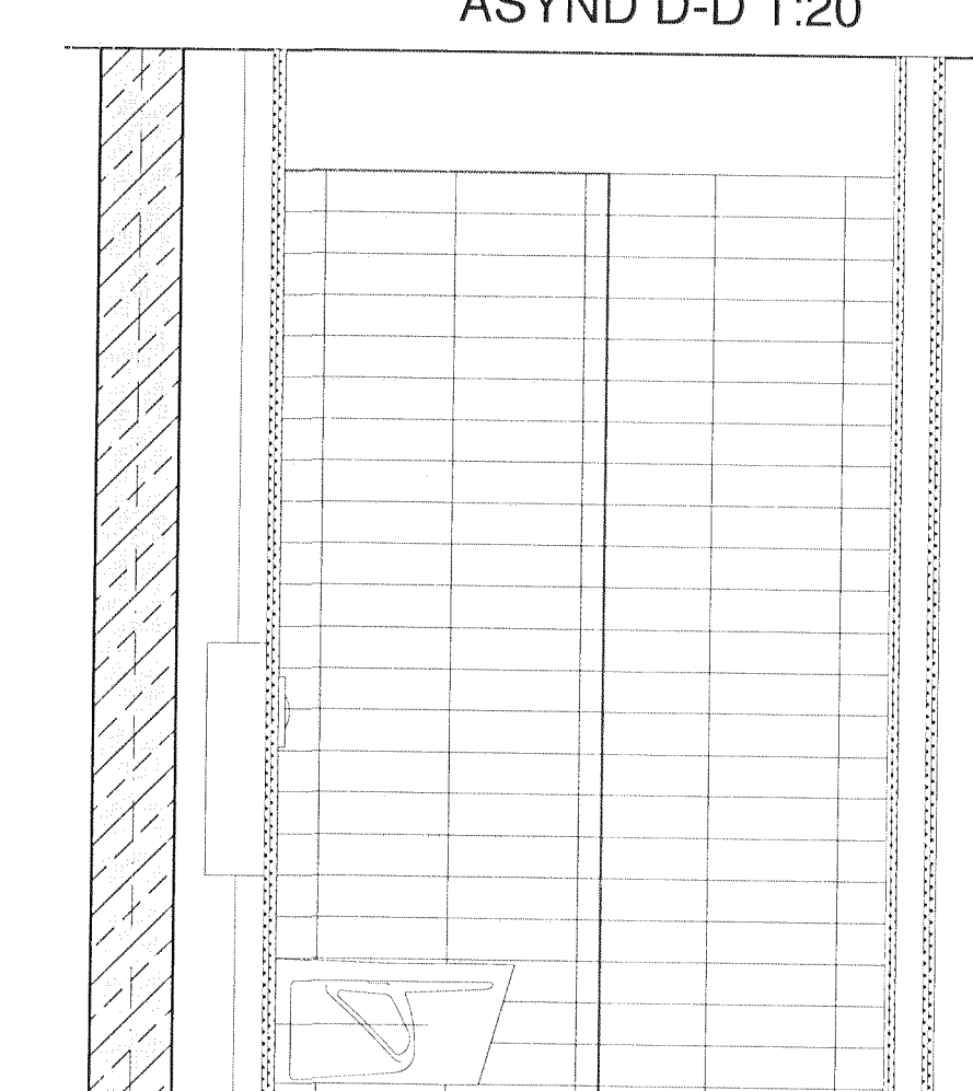
ÁSÝND B-B 1:20
