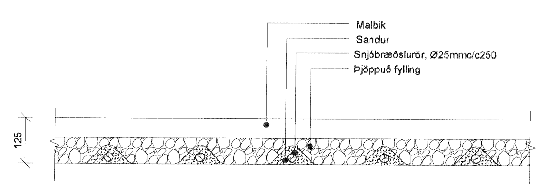
KENNISNIÐ SNJÓBRÆÐSLU Í MALBIK 1:10
