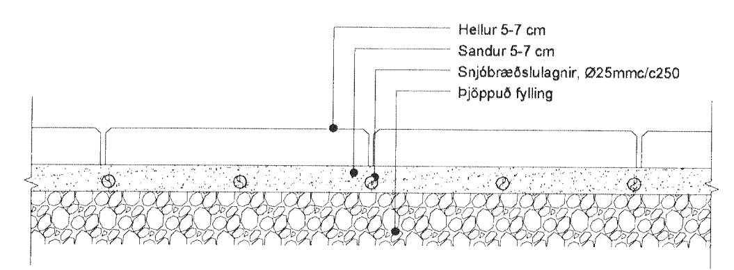
KENNISNIÐ SNJÓBRÆÐSLU Í HELLUR 1:10
