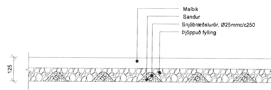
KENNISNIÐ SNJÓBRÆÐSLU Í MALBIK 1:10
