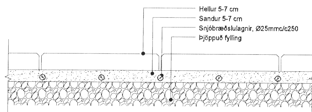
KENNISNIÐ SNJÓBRÆÐSLU Í HELLUR 1:10
