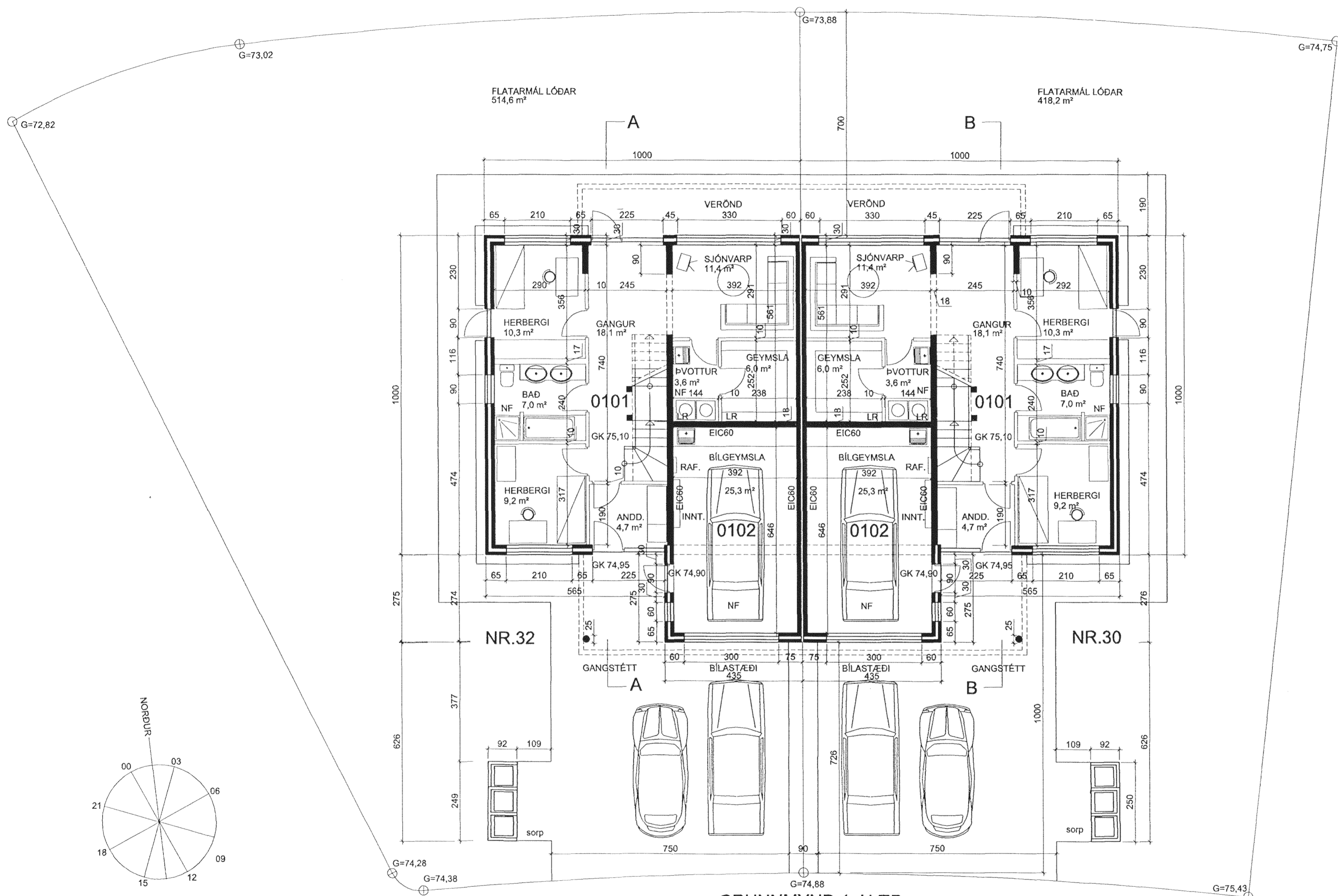
GRUNNMYND 1. HÆÐ
