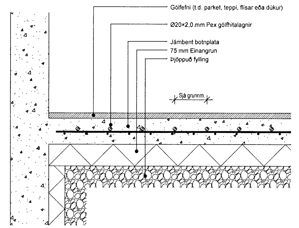
KENNISNIÐ GÓLFHITA 1:10
